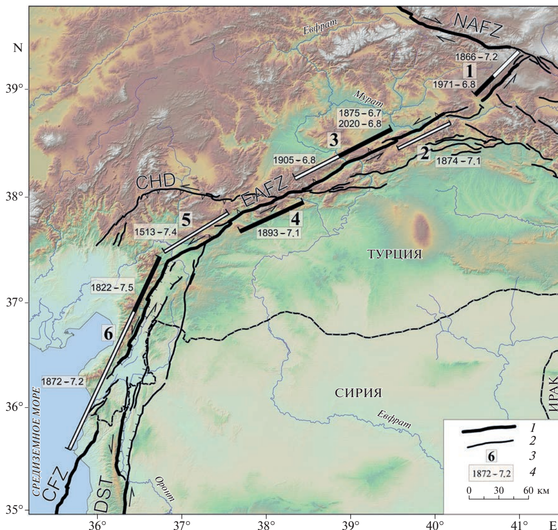
Рис. 4. Сеймотектоническая сегментация EAFZ. Сегментация выполнена по работе [Duman, Emre, 2013] с изменениями; данные о землетрясениях почерпнуты из работ [Ambraseys, 1989; Ambraseys, Jackson, 1998], активные разломы Сирии и северного продолжения DST в Турции изображены по работе [Trifonov, 2012]. Цифрами обозначены сегменты: 1 – Карлиова–Бингёль; 2 – Палу–оз. Хазар; 3 – оз. Хазар–Синджик; 4 – Челикхан–Эркенек; 5 – Гельбаши–Тюркоглу; 6 – Тюркоглу–Антакия.
