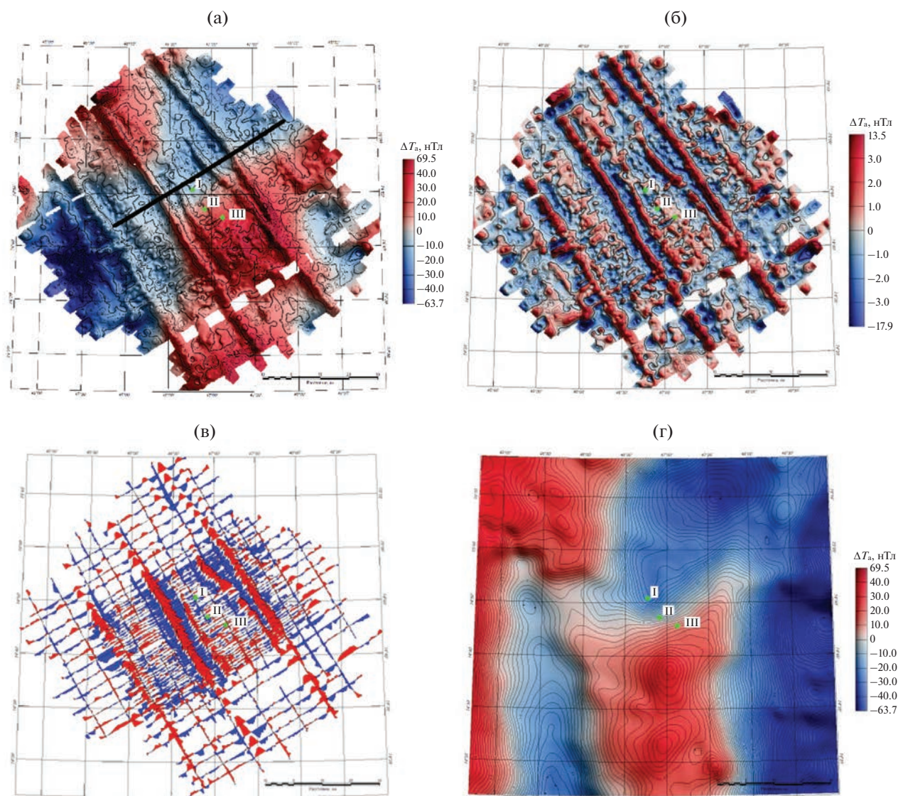
Рис. 6. Сопоставление результатов гидро- и аэромагнитной съемки, выполненных на Лудловской площади, расположенной в глубоководной части акватории Баренцева моря. Гидромагнитная съемка: исходное anomальное магнитное поле (а); локальная компонента anomального магнитного поля (период среза 10 км) (б); карта-графиков локальной аномалий (ФВЧ 10 км) (в). Аэромагнитная съемка: anomальное магнитное поле (г). Римскими цифрами I, II, III отмечено местоположение скважин Лудловская-1, Лудловская-2, Лудловская-3. Линия черного цвета на фрагменте (а) — профиль оценок параметров источников магнитных аномалий (результаты оценок см. ниже в разделе Заключение).
