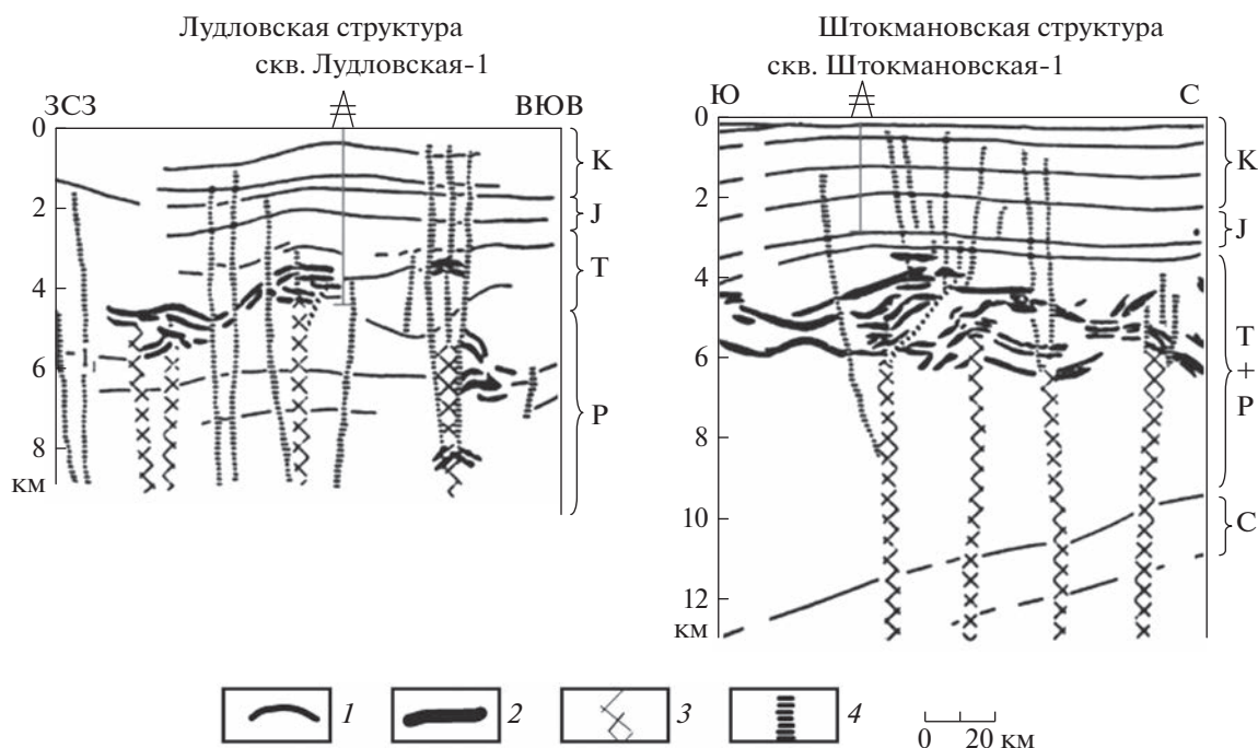
Рис. 1. Геолого-геофизические разрезы Лудловской и Штокмановской структур (по работе [Шипилов, Юнов, 1995] с изменениями). Условные обозначения: 1 — основные опорные отражающие горизонты в осадочном чехле; 2 — силлы долеритов (изображены вне масштаба); 3 — магмоподводящие каналы; 4 — разломы. Над разрезом отмечено положение скважин, упоминаемых в тексте; справа от разрезов указан возраст толщ осадочного чехла.
