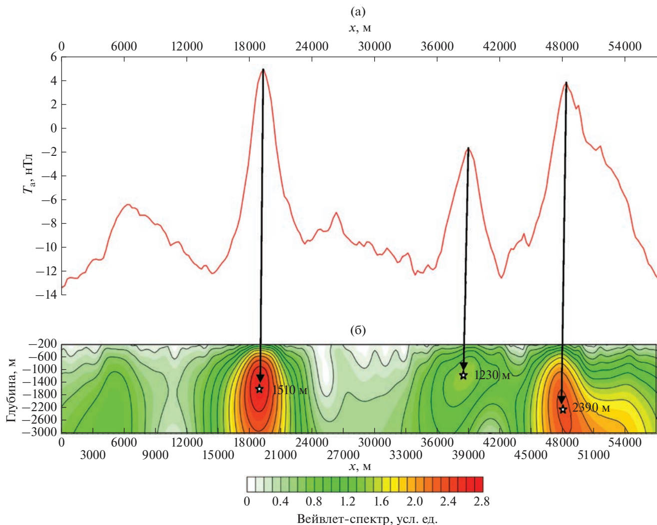
Рис. 8. Оценка параметров источников магнитных линейных аномалий на одном из профилей Лудловской площади (положение профиля см. на рис. 6а): (а) — графики аномального магнитного поля; (б) — вейвлет-спектр, полученный вейвлетами Пуассона первого порядка с масштабным коэффициентом второго порядка 1/h , сечение изолиний 0.1 усл. ед.
