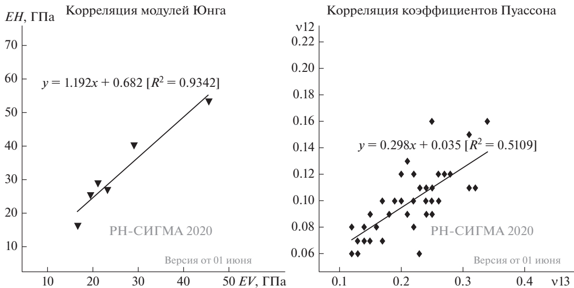
Рис. 2. Результаты керновых исследований по определению модулей упругости бажендовской свиты.
