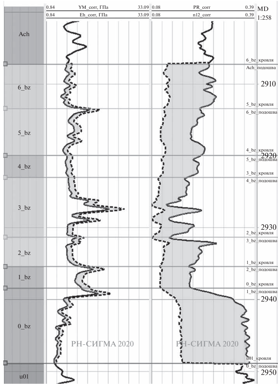
Рис. 3. Профили упругих модулей трансверсально-изотропной среды. Левый трек содержит модули Юнга, правый – коэффициенты Пуассона. Сплошными линиями обозначены модули при нагружении поперек напластования ( E_V , \nu_{31} ), а пунктиром – модули при нагружении вдоль напластования ( E_H , \nu_{12} ).
