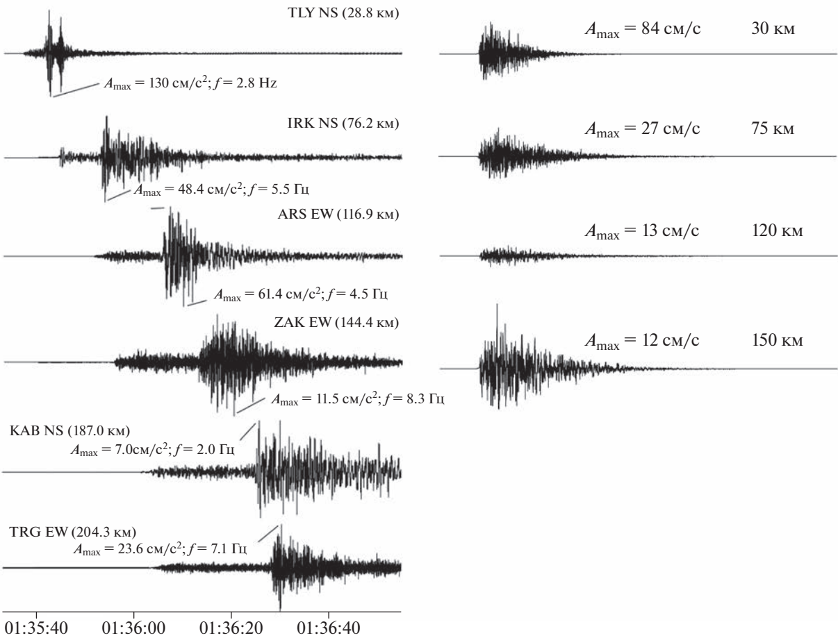
Рис. 5. Акселерограммы Култуковского землетрясения (из работы [Мельникова и др., 2014]) в сравнении с акселерограммами, построенными в настоящей работе. Горизонтальные и вертикальные оси имеют один масштаб для акселерограмм, расположенных на одном уровне по горизонтали.
