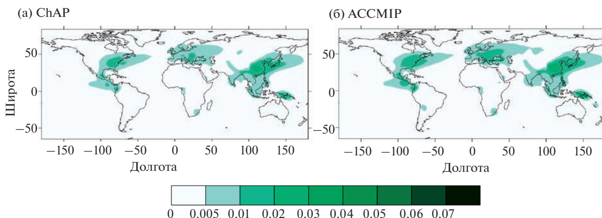
Рис. 1. Влажное осаждение \text{SO}_x ( \text{MrS m}^{-2} \text{год}^{-1} ) для 2000 г. по расчетам со схемой ChAP (а; учитывается только влажное осаждение \text{SO}_4 ) и по результатам проекта ACCMIP [25] (б).
