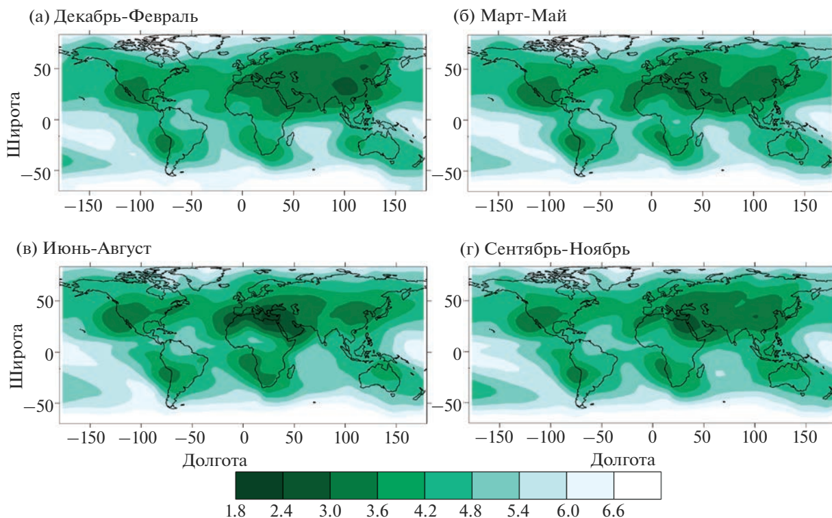
Рис. 4. Подобно рис. 2, но для эмиссий соединений серы в атмосферу, соответствующих 2000 г.
