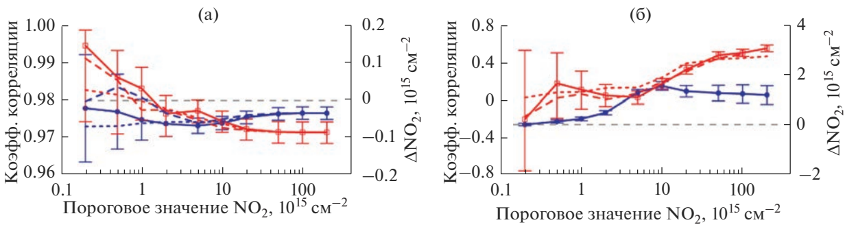
Рис. 10. Коэффициент корреляции (красный цвет) и средняя разность (синий цвет) между значениями содержания NO 2 в столбе стратосферы (а) и тропосферы (б) по данным ОМІ и данным наземных измерений на ЗНС в зависимости от верхнего порогового значения содержания NO 2 в столбе тропосферы. Пороговое значение применялось одновременно к данным ОМІ и данным ЗНС (сплошные кривые), только к данным ОМІ (штриховые кривые) или только к данным ЗНС (пунктирные кривые).
