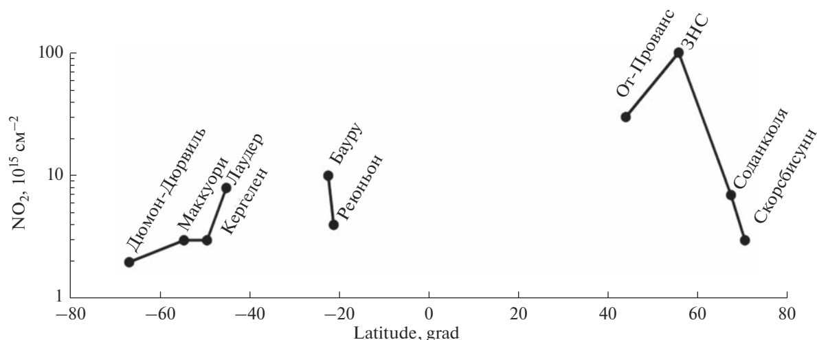
Рис. 11. Широтная зависимость максимального порогового значения содержания NO_2 в столбе тропосферы в окрестностях станций NDACC по данным OMI.
