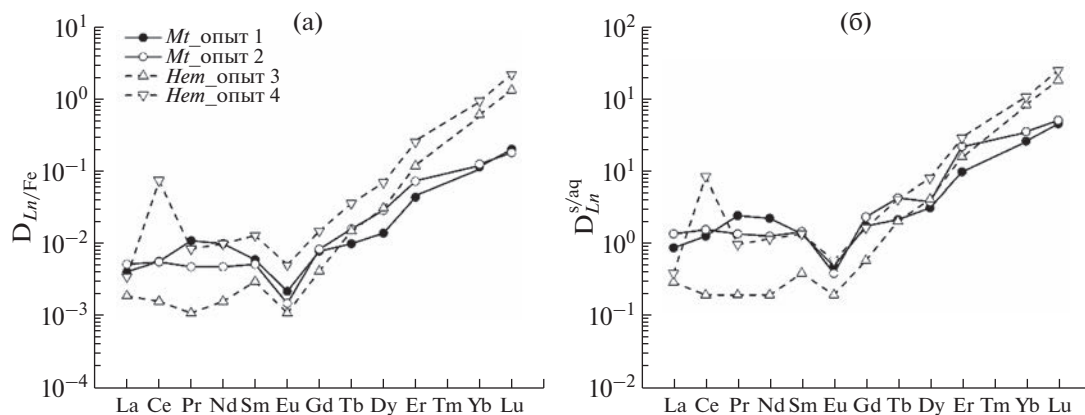
Рис. 5. Результаты экспериментов по распределению Ln между магнетитом ( Mt ), гематитом ( Hem ) и гидротермальным раствором при 450 °С и давлении 1 кбар.
