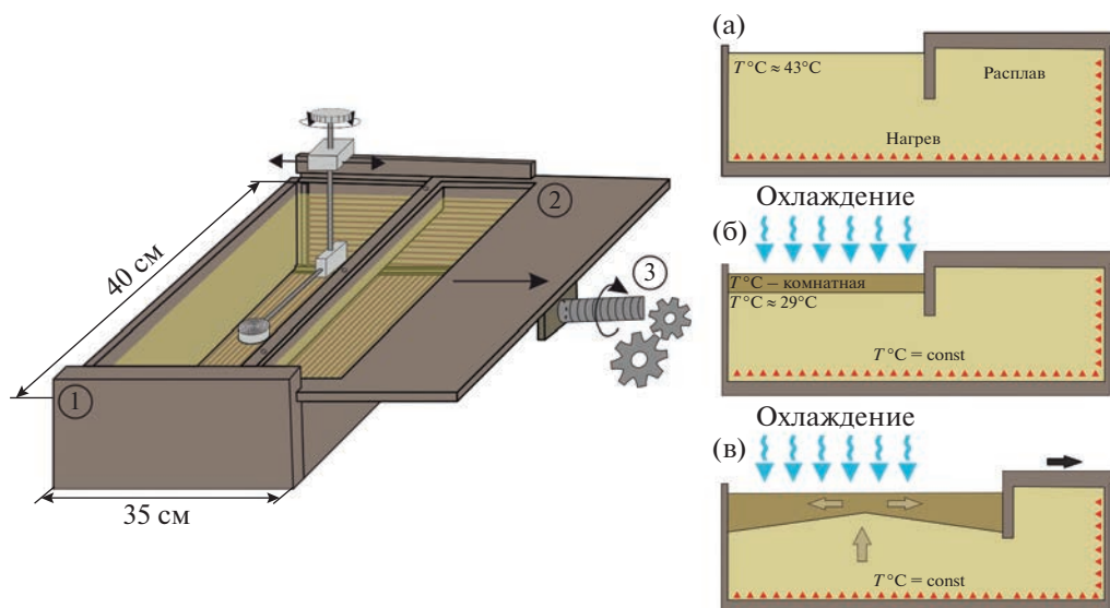
Рис. 4. Экспериментальная установка (слева), подготовка модели в разрезе (справа).
