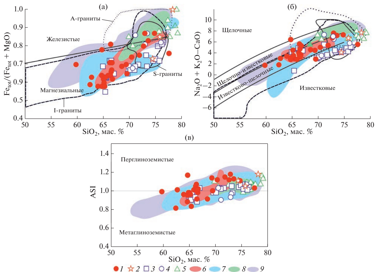
Рис. 9. (а) Диаграммы \text{Fe}_{\text{tot}}/(\text{Fe}_{\text{tot}} + \text{MgO}) — \text{SiO}_2 , (б) \text{Na}_2\text{O} + \text{K}_2\text{O} - \text{CaO} — \text{SiO}_2 , (в) \text{ASI} — \text{SiO}_2 [29] для гранитоидов Эликчанского, Куранахского и Бакинского массивов Северного вулcano-плутонического пояса 1–2 – гранитоиды Эликчанского массива: 1 – 1-ой фазы, 2 – даек 2-ой фазы; 3–4 – гранитоиды Куранахского массива: 3 – 1-ой фазы, 4 – даек 2-ой фазы; 5 – граниты, лейкограниты Бакинского массива; 6–9 – поля гранитоидов массивов: 6 – Эликчанского, по [21, 37], 7 – Куранахского, по [21, 37]; 8 – Бакинского, по [21]; 9 – Улахан-Тас Северного пояса, по [2]
