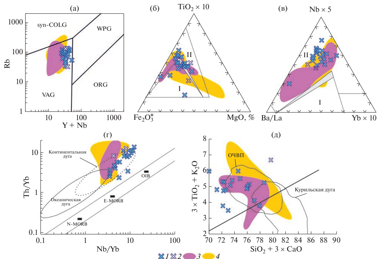
Рис. 14. Диаграммы (а) Rb-(Y + Nb) [36], (б) Fe_2O_3^*-TiO_2 \times 10-MgO , (в) Ba/La-Nb \times 5-Yb \times 10 [31], (г) Th/Yb-Nb/Yb [35] и (д) 3 \times TiO_2 + K_2O-SiO_2 + 3 \times CaO [14] для вулканитов тумусской толщи и субвулканических тел тумусского комплекса. 1 – вулканиты тумусской толщи; 2 – субвулканические тела тумусского комплекса; 3–4 – вулканиты впадин: 3 – Тытельвеемской [19], 4 – Тытельвеемской [25]
