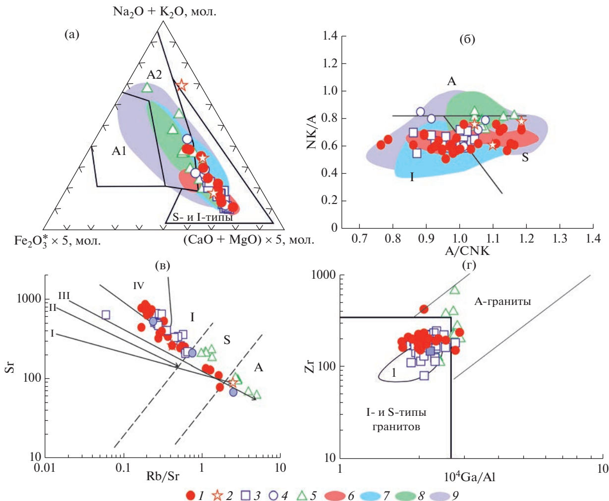
Рис. 11. Диаграммы (а) \text{Fe}_2\text{O}_3^* \times 5 - \text{Na}_2\text{O} + \text{K}_2\text{O} - (\text{CaO} + \text{MgO}) \times 5 ( \text{SiO}_2 > 67\% , мол. кол-ва) [5], (б) \text{NK/A} - \text{A/CNK} [34], (в) \text{Sr} - \text{Rb/Sr} [6] и (г) \text{Zr} - 10^4 \text{Ga/Al} [39] для гранитоидов Эликчанского, Куранахского и Бакынского массивов Северного вулcano-плутонического пояса.
