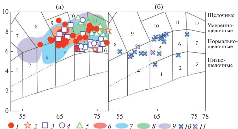
Рис. 8. (а) Диаграммы TAS [23] для гранитоидов Эликчанского, Куранахского и Бакынского массивов и (б) вулканитов и даек тумусского комплекса Северного вулcano-плутонического пояса.
