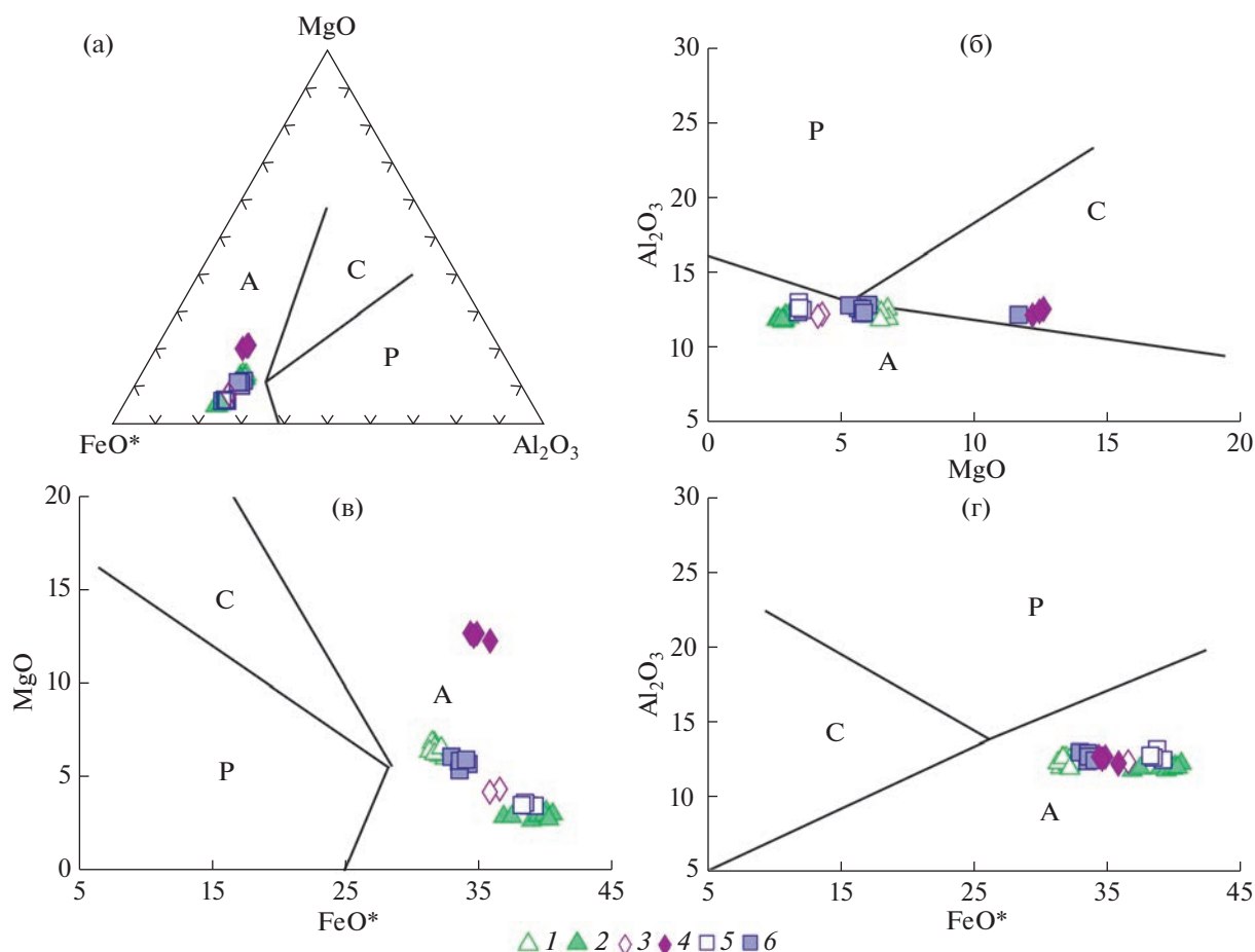
Рис. 15. Диаграммы (а) \text{FeO}^*\text{--MgO--Al}_2\text{O}_3 , (б) \text{Al}_2\text{O}_3\text{--MgO} , (в) \text{MgO--FeO}^* и (г) \text{Al}_2\text{O}_3\text{--FeO}^* [24] для биотитов из гранитоидов Бакынского массива. Поля биотитов из: А – анорогенных щелочных гранитоидов, Р – пералюминиевых гранитоидов, включая S-тип, С – из известково-щелочных гранитоидов.
