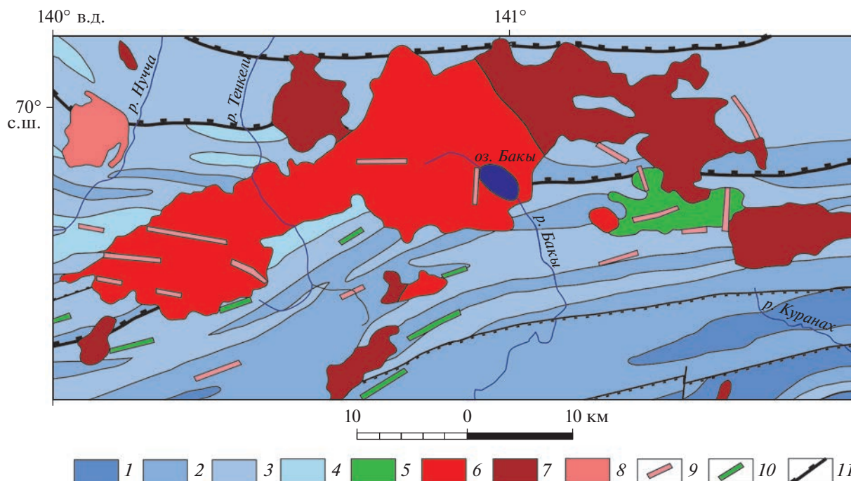
Рис. 5. Геологическая карта Бакинского массива.
