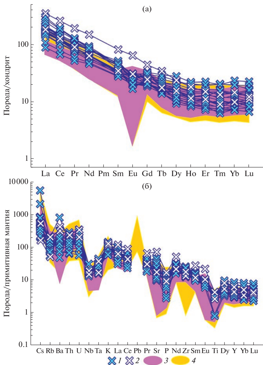
Рис. 13. Хондрит-нормализованные распределения РЗЭ (а) и спайдерграммы редких элементов, нормированных на состав примитивной мантии (б) для вулканитов тумусской толщи и субвулканических тел тумусского комплекса. 1 – вулканиты тумусской толщи; 2 – субвулканические тела тумусского комплекса; 3–4 – вулканиты впадин: Тытельвеевской [19], 4 – Тытельвеевской [25]
