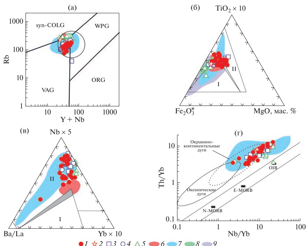
Рис. 12. Диаграммы (а) Rb—(Y + Nb) [35], (б) \text{Fe}_2\text{O}_3^* — \text{TiO}_2 \times 10 —MgO, (в) Ba/La—Nb \times 5 —Yb \times 10 [31], (г) Th/Yb—Nb/Yb [35] для гранитоидов Эликчанского, Куранахского и Бакынского массивов Северного вулканно-плутонического пояса. Обозначено на (б)—(в) — поля магматических пород: I — островные дуги и континентальные окраины (конвергентные окраины); II — границ скольжения (трансформные окраины континентов и островных дуг). 1—2 — гранитоиды Эликчанского массива: 1 — 1-ой фазы, 2 — даек 2-ой фазы; 3—4 — гранитоиды Куранахского массива: 3 — 1-ой фазы, 4 — даек 2-ой фазы; 5 — граниты, лейкограниты Бакынского массива; 6—9 — поля гранитоидов массивов: 6 — Эликчанского, по [21, 37], 7 — Куранахского, по [21, 37], 8 — Бакынского, по [21], 9 — Улахан-Тас Северного пояса, по [2]
