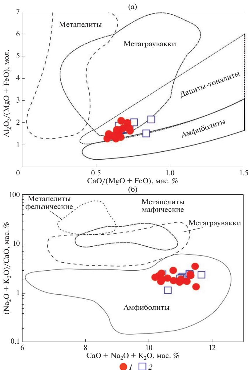
Рис. 16. Диаграммы (а) \text{Al}_2\text{O}_3/(\text{MgO} + \text{FeO}) – \text{CaO}/(\text{MgO} + \text{FeO}) мол. кол-ва [30] и (б) (\text{Na}_2\text{O} + \text{K}_2\text{O})/\text{CaO} – \text{CaO} + \text{Na}_2\text{O} + \text{K}_2\text{O} [26] мас. % для гранитоидов Эликчанского, Куранахского и Бакынского массивов Северного вулcano-плутонического пояса.
