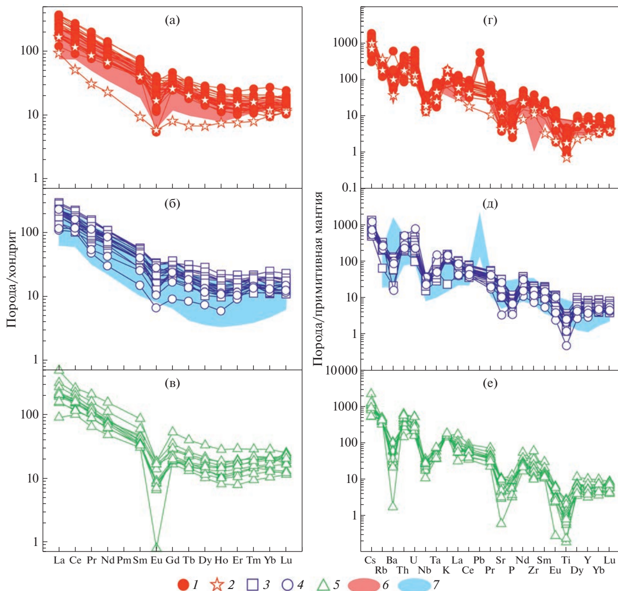
Рис. 10. Хондрит-нормализованные распределения РЗЭ (а–в) и спайдерграммы редких элементов, нормированных на состав примитивной мантии (г–е) гранитоидов Эликчанского, Куранахского и Бакинского массивов Северного вулканно-плутонического пояса.
