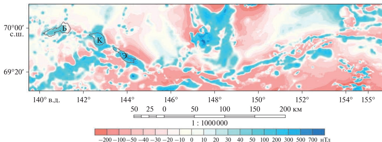
Рис. 4. Карта аномального магнитного поля ( \Delta T_a ).
