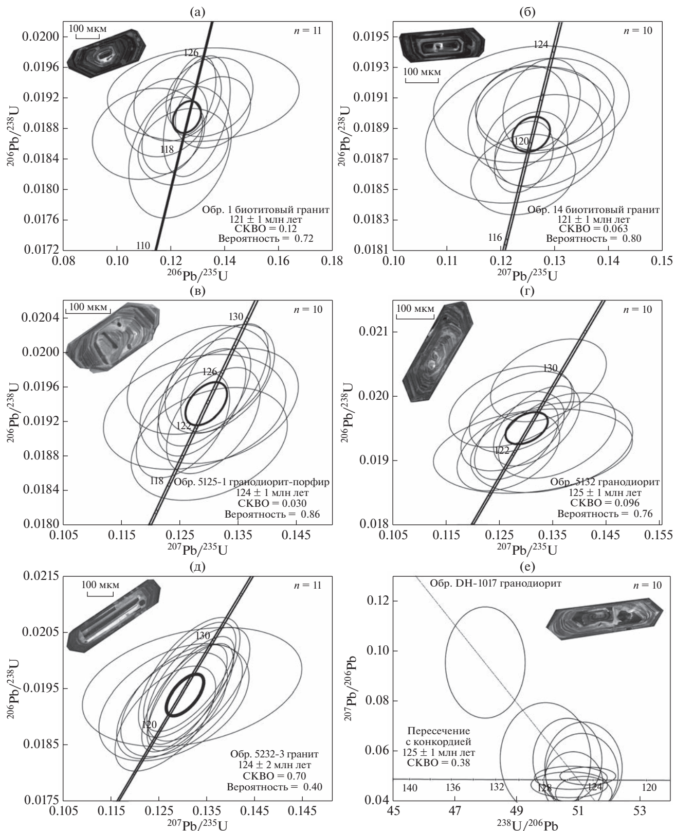
Рис. 6. Диаграммы с конкордией (U–Pb SIMS) и микрофотографии цирконов в режиме катодолюминисценции. (а)–(б) – для биотитовых гранитов (обр. № 1, № 14) Бакынского массива; (в)–(г) – для гранодиорит-порфира и гранодиорита 1-ой фазы (обр. № 5125-1, № 5132) Эликчанского массива; (д)–(е) – для гранодиорита 1-ой фазы, пегматитового гранита 2-ой фазы (№ DH-1017, обр. № 5132-3), Куранахского массива.
