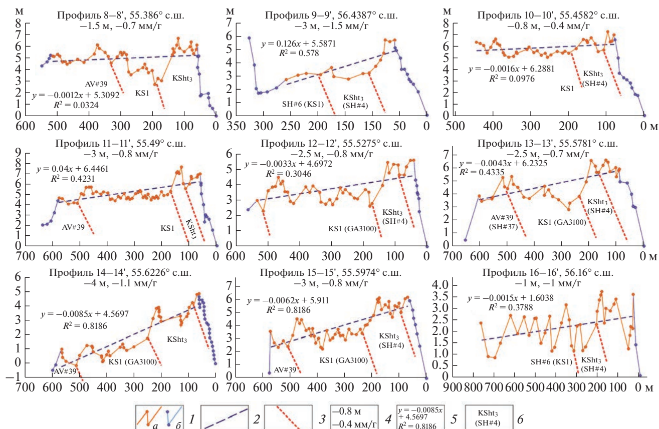
Рис. 6. Профили 8–8'–16–16' через опускающееся побережье Камчатского залива.
