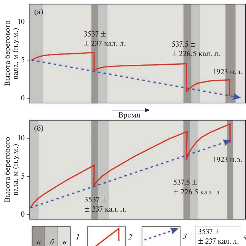
Рис. 9. Схема сейсмических циклов и косейсмических опусканий побережья Камчатского залива во время сильных субдукционных землетрясений (по данным [15], с изменениями). Части Камчатского залива: (а) — центральная, (б) — южная. 1 — вертикальные движения в пределах цикла: а — косейсмическое, б — быстрое постсейсмическое, в — медленное интерсейсмическое; 2 — высота древнейшего берегового вала на протяжении нескольких сейсмических циклов; 3 — тренд вертикальных движений побережья; 4 — средневзвешенное значение возраста установленных событий (калиброванных лет до 1950 г.)
