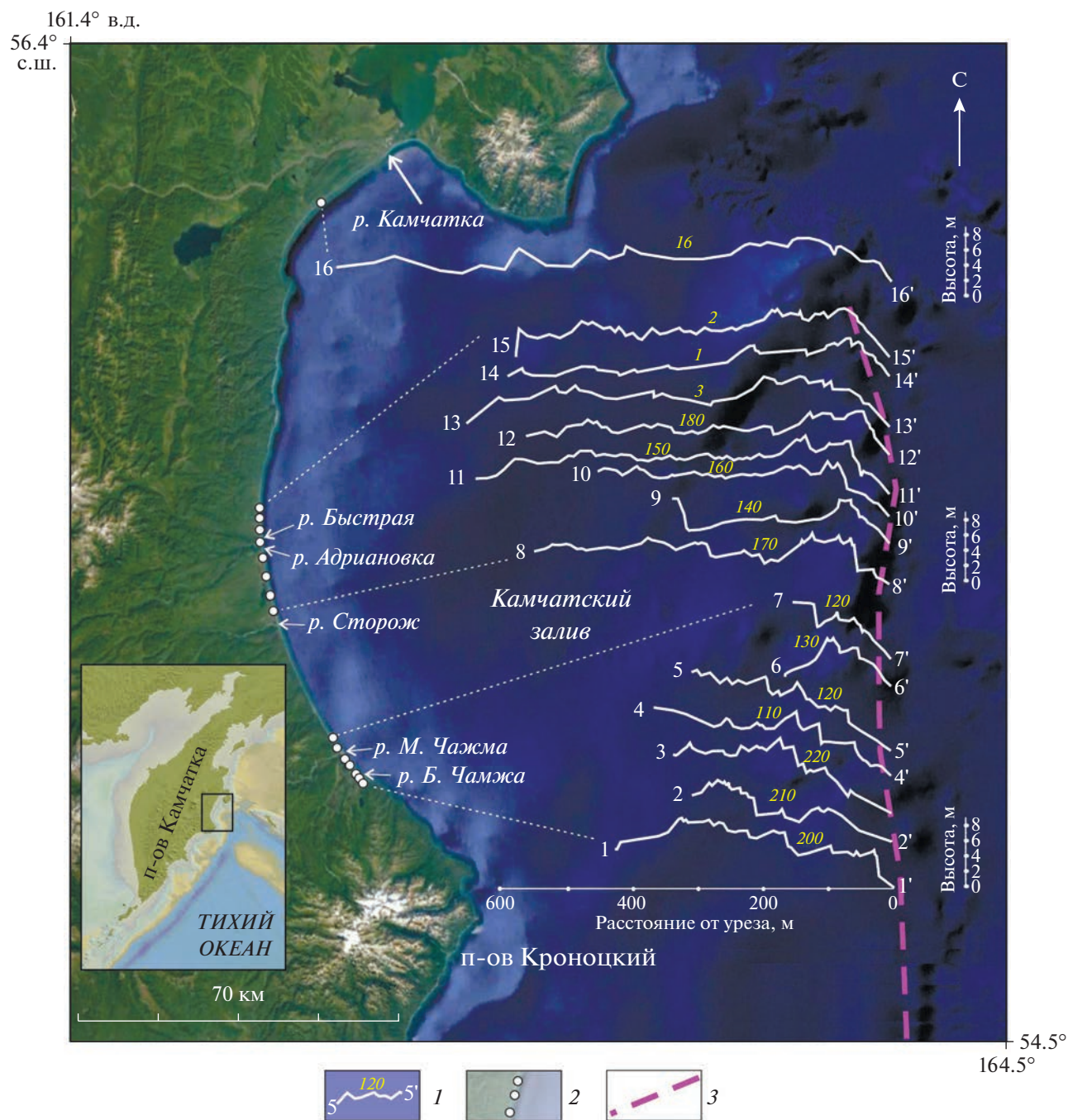
Рис. 3. Измеренные топографические профили 1–1'–16–16' на побережье Камчатского залива (по [29]).
