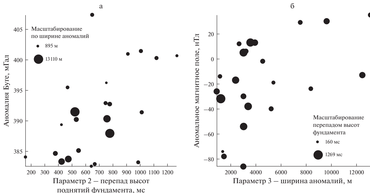
Рис. 7. Кросс-корреляция значений геофизических полей и морфометрических параметров аномалий “плоское пятно”. а — аномалии Буге, по [Balmino et al., 2012], и перепад высот поднятий фундамента; б — аномальное магнитное поле \Delta T_a , по [Maus et al., 2009], и ширина плоских пятен. Здесь и на рис. 8 линейное масштабирование символов сделано по параметру 3 (для а — ширина аномалии) и параметру 2 (для б — перепад высот фундамента). Минимальные и максимальные размеры символов (черные кружки) имеют условные значения.
