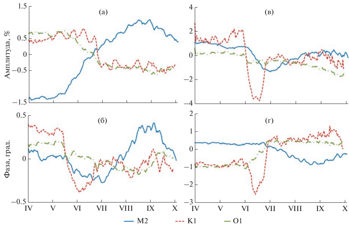
Рис. 4. Ход отклонений амплитуд и фаз волн M2, K1 и O1 за расчетный период: (а, б) – пост м. Тайгонос; (в, г) – пост б. Причальная за безледный период.
