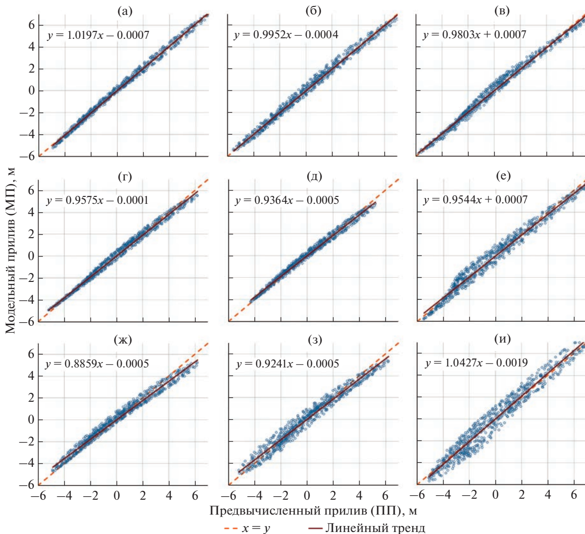
Рис. 2. Корреляционные диаграммы модельного и предвычисленного приливного уровня моря для постов в акватории Пенжинской губы: о. Ивиньчаман (а), м. Рифовый (б), м. Водопадный (в), м. Средний (г), м. Тайгонос (д), м. Угольный (е), р. Яваям (ж), б. Причальная (з), м. Астрономический (и).
