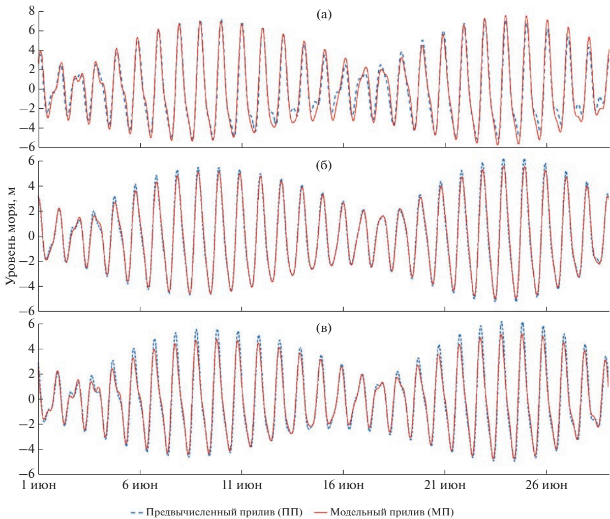
Рис. 5. График МП и ПП для постов с различными оценками моделирования: (а) м. Астрономический; (б) м. Средний; (в) м. Яваям.
