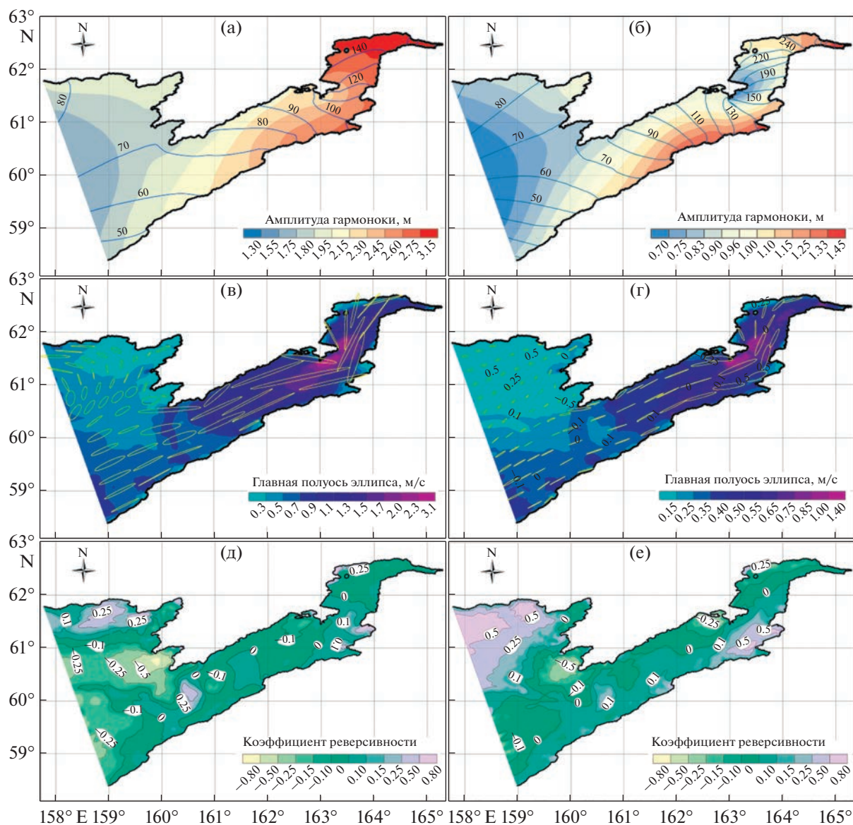
Рис. 3. Характеристики амплитуд и поверхностных течений основных волн прилива: (а) — котидальная карта амплитудных характеристик приливной “лунной-солнечной деклинационной, суточной” волны K1, (б) — котидальная карта амплитудных характеристик “главной лунной полусуточной” волны M2, (в) — приливные эллипсы волны K1, (г) — приливные эллипсы волны M2, (д) — пространственное распределение коэффициента реверсивности приливного эллипса и его полярность для суточной волны K1, (е) — пространственное распределение коэффициента реверсивности приливного эллипса волны M2.
