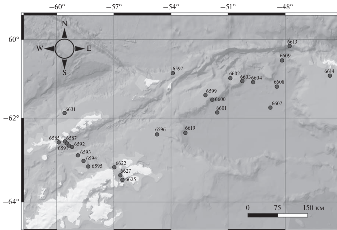
Рис. 1. Карта станций 79 рейса НИС «Академик Мстислав Келдыш» в водах Атлантического сектора Антарктики, 11 января–4 февраля 2020 г.
