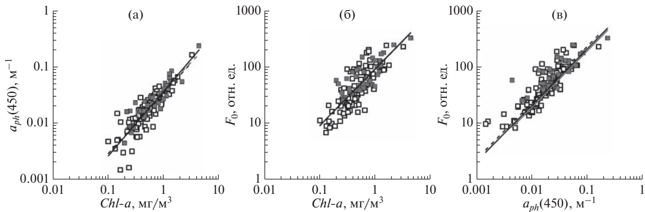
Рис. 4. (а) – Связь показателя поглощения света пигментами фитопланктона на длине волны 450 нм ( a_{ph}(450) ) с концентрацией хлорофилла а ( Chl-a ) в выбранных слоях; (б) – связь интенсивности флуоресценции, регистрируемой лабораторным флуориметром после темновой адаптации ( F_0 ) с Chl-a в выбранных слоях; (в) – связь F_0 с a_{ph}(450) в выбранных слоях исследуемой акватории в водах Атлантического сектора Антарктики, 11 января–4 февраля 2020 г., обозначения см. на рис. 2.
