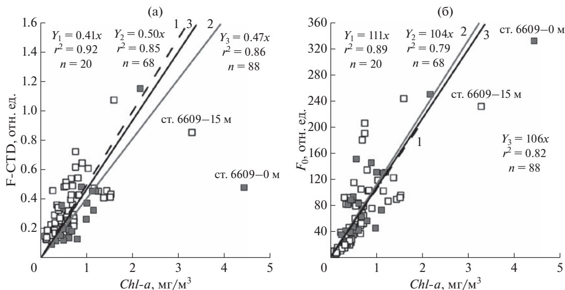
Рис. 3. Связь интенсивности флуоресценции хлорофилла a измеренной погружным датчиком (а) и на лабораторном флуориметре (б) с концентрацией хлорофилла a , измеренной спектрофотометрическим методом, в различных оптических слоях исследуемой акватории в водах Атлантического сектора Антарктики, 11 января–4 февраля 2020 г., обозначения см. на рис. 2.
