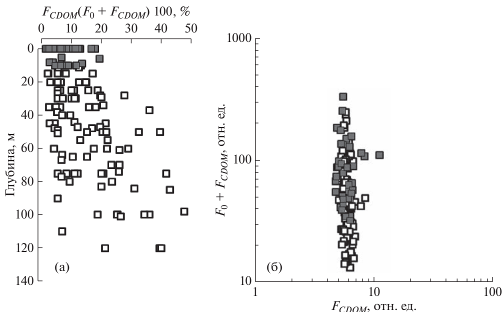
Рис. 2. (а) — Изменение относительного вклада флуоресценции растворенного органического вещества ( F_{CDOM} ) в общую флуоресценцию ( F_{CDOM} + F_0 ) по глубине во всей исследуемой акватории; (б) — изменение абсолютных величин F_{CDOM} + F_0 в зависимости от величины F_{CDOM} в различных оптических слоях (■ — глубины \leq 1 оптической глубины; □ — глубины > 1 оптической глубины) исследуемой акватории в водах Атлантического сектора Антарктики, 11 января—4 февраля 2020 г.
