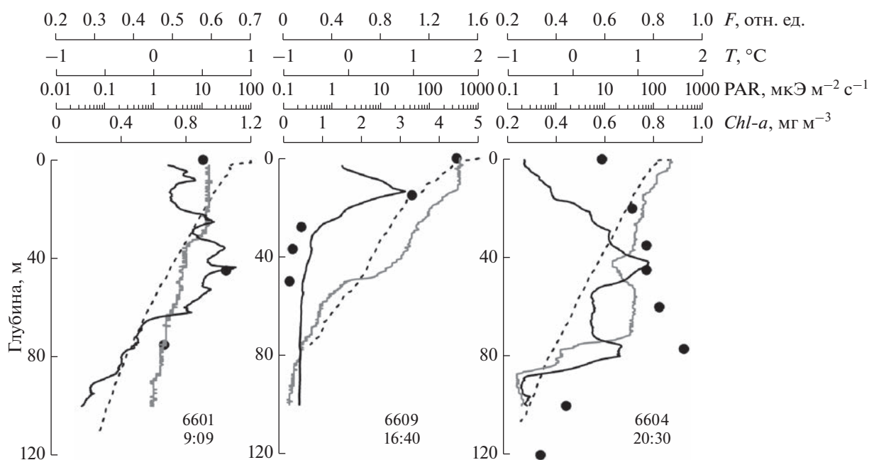
Рис. 5. Профили вертикального распределения: температуры ( T ) — серая линия; интенсивности PAR, измеренной Li-COR — пунктирная линия; интенсивности флуоресценции ( F ) измеренной погружным датчиком ПУМ-200 — черная линия, и концентрации хлорофилла a ( Chl-a ) — ● на отдельных станциях в слоях в водах Атлантического сектора Антарктики, 11 января—4 февраля 2020 г., обозначения см. рис. 2.
