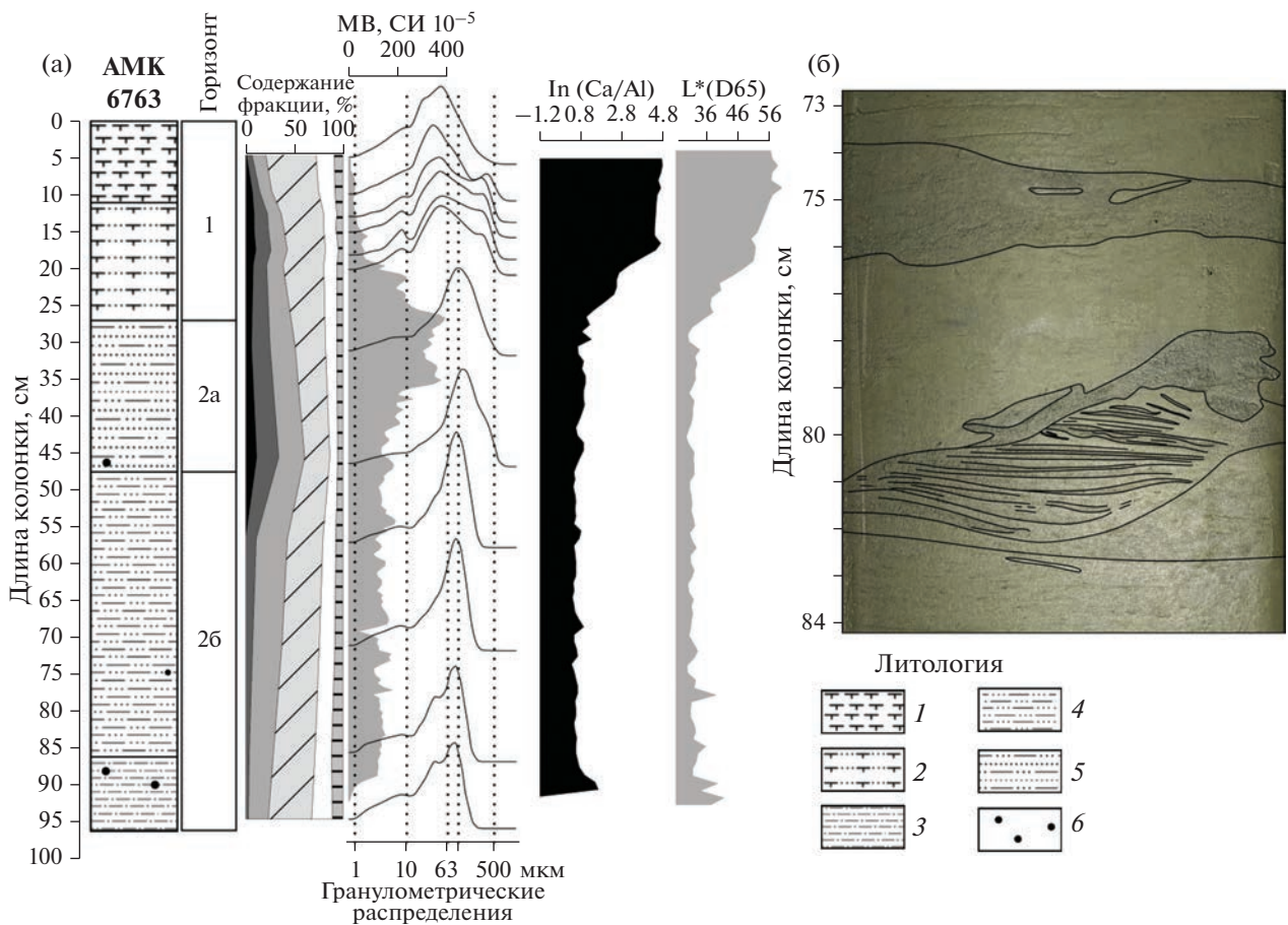
Рис. 4. Колонка АМК-6763. а – Литология, гранулометрия, магнитная восприимчивость (МВ), отношение Ca/Al, уровень яркости цвета осадков (L*). б – Фрагмент фотографии колонки с линзами, указывающими на контуритовую природу осадков. Условные знаки: Гранулометрия – см. рис. 3. Литология: 1 – известковый песок, сiltистый песок, песчаный сilt; 2 – песчаный сilt терригенно-известковый; 3 – сilt терригенный; 4 – песчаный сilt терригенный; 5 – сiltистый песок терригенный; 6 – галька и гравий.
