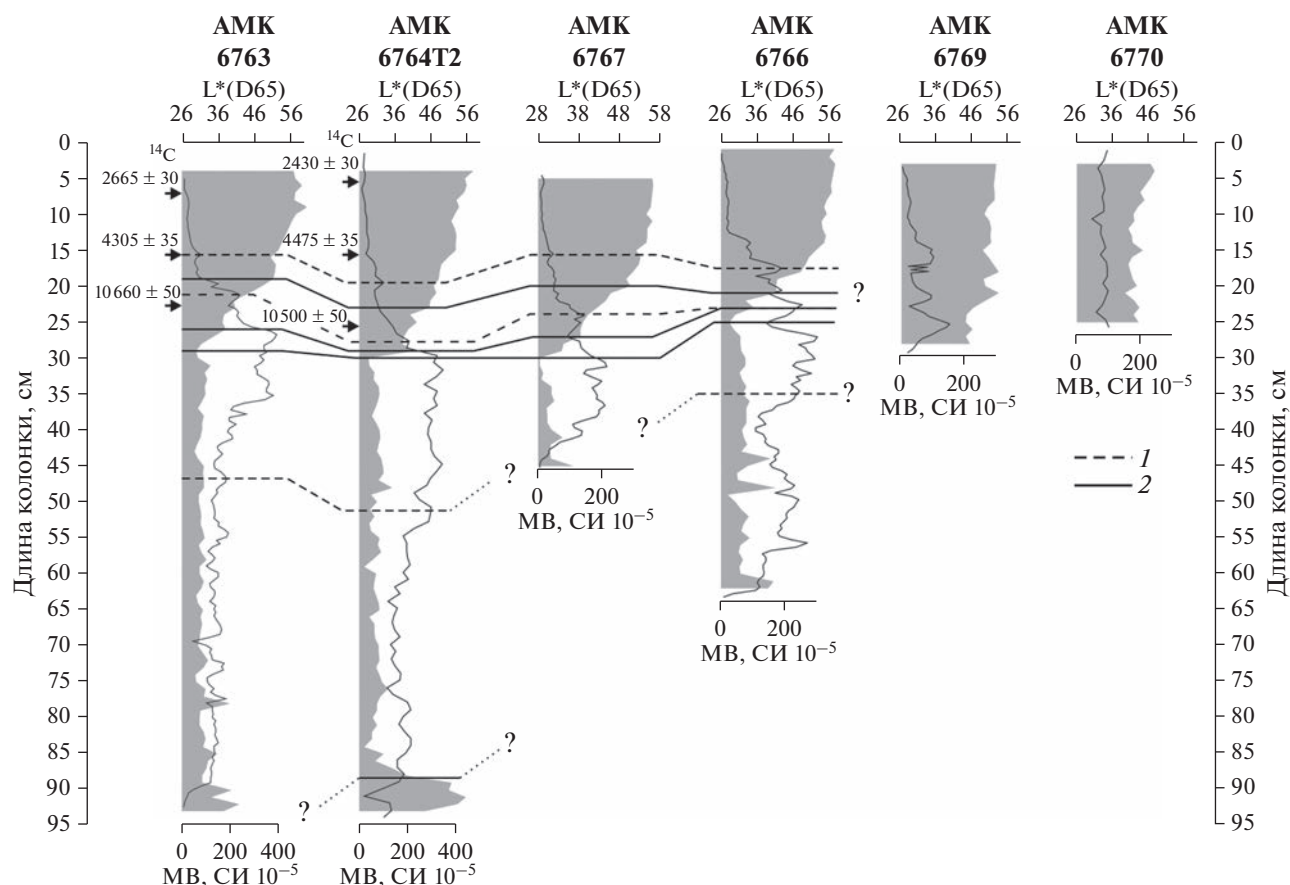
Рис. 5. Магнитная восприимчивость (МВ), уровень яркости цвета осадков (L*), масс-спектрометрические радиоуглеродные датировки и корреляция колонок сектора Амегино. 1 — корреляция пиков МВ, 2 — корреляция пиков уровня яркости (L*).
