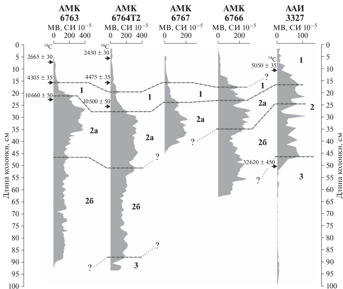
Рис. 7. Удаленная лито- хроностратиграфическая корреляция 4 колонок сектора Амегино и террасы Пьедра Буэна (АИ-3327) с учетом масс-спектрометрических радиоуглеродных датировок и изменений магнитной восприимчивости (МВ).
