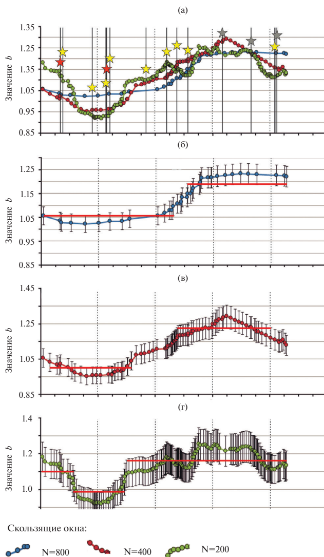
Рис. 5. Временной ход наклона графика повторяемости (здесь значение b \equiv b^{mb} ), рассчитанный в скользящих окнах шириной N = 800, 400, 200 землетрясений; вертикальные полосы – момент возникновения сильных землетрясений с m_b \geq 6.5 (а). Временной ход наклона графика повторяемости (значение b ), рассчитанный в скользящих окнах разной ширины; вертикальные отрезки – стандартное отклонение значения b ; красная горизонтальная линия – временной интервал, в пределах которого значение b постоянно (б–г).
