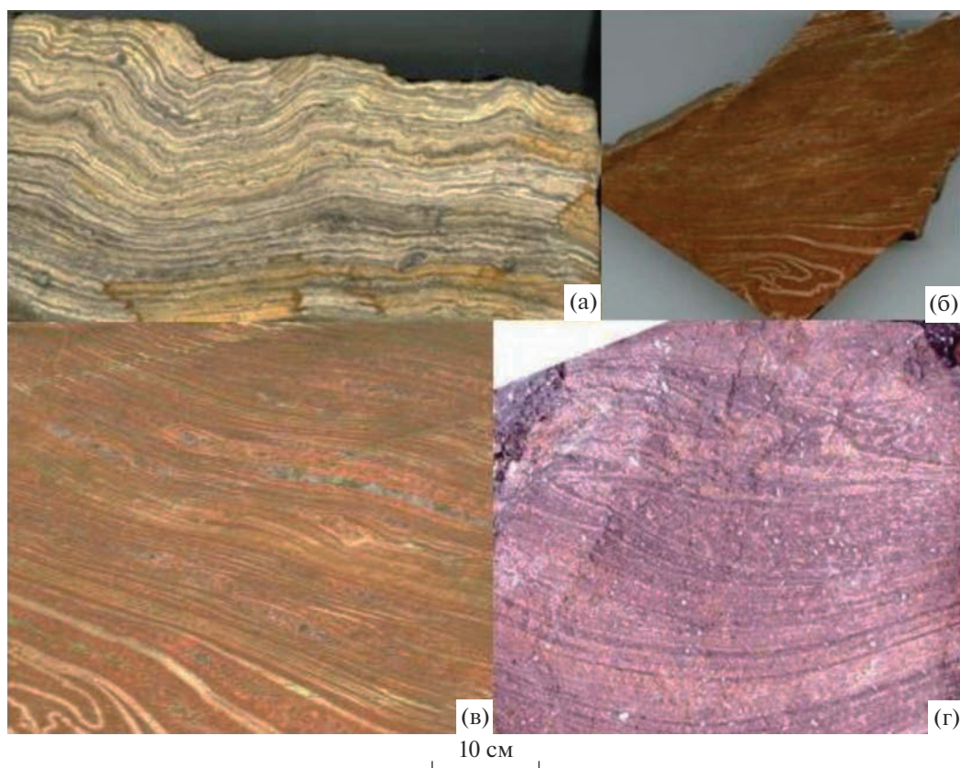
Рис. 3. Флюидално-полосчатые кремнекислые лавы разных регионов.
