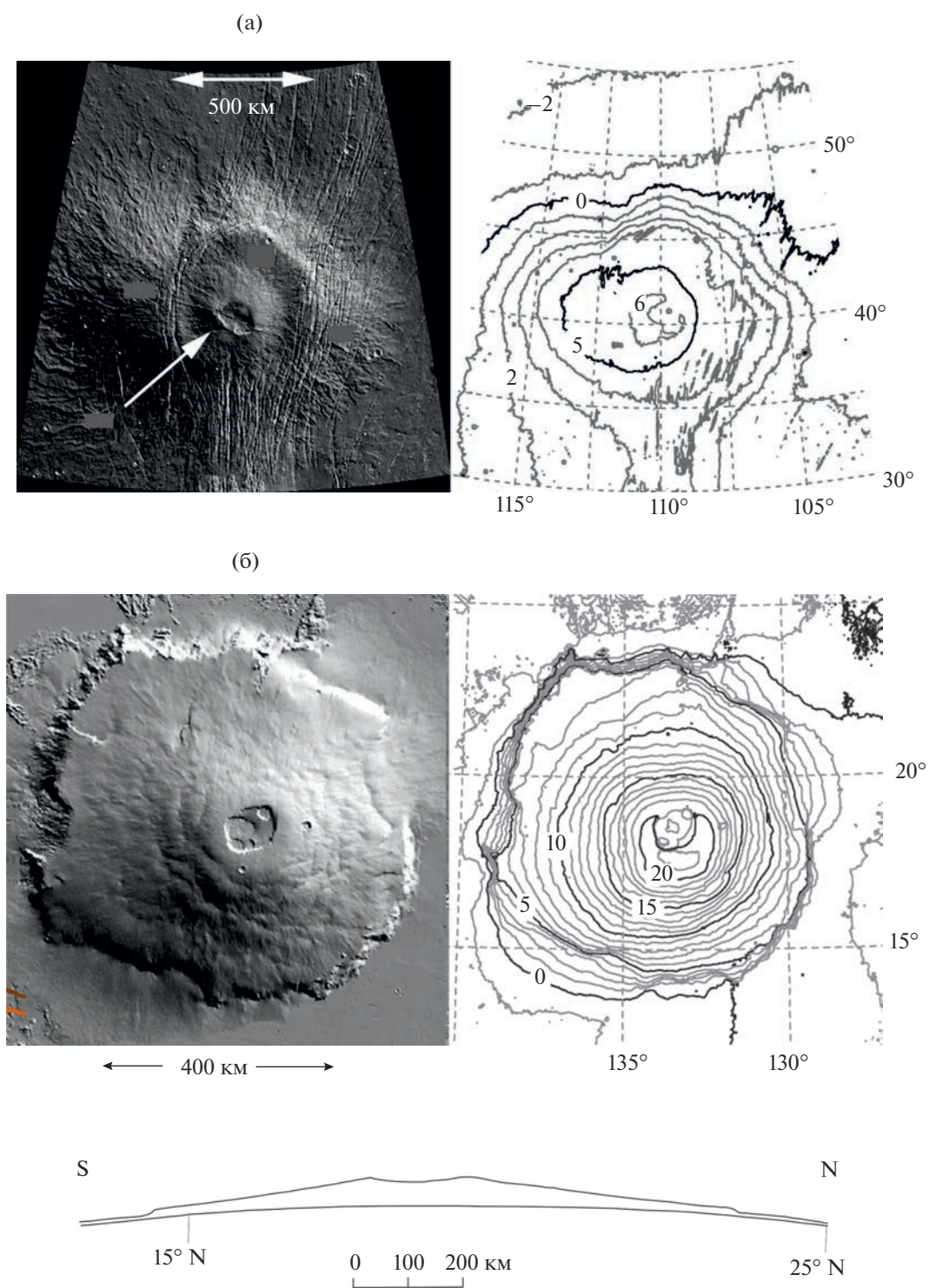
Рис. 2. Космические изображения и карты МГС патера Альба (а) и г. Олимп (б) с поперечным профилем. Горизонталы обычные проведены через 1 км, утолщенные — через 5 км. На патере Альба стрелкой показан кальдерный комплекс размером 106 \times 138 км. Видны субмеридиональные и дугообразные разрывные нарушения над кровлей магматического суперпотока (см. рис. 1). На г. Олимп освещенный с СВ круговой уступ имеет высоту 3–6 км, а размер вершинного кальдерного комплекса — 72 \times 91 км.
