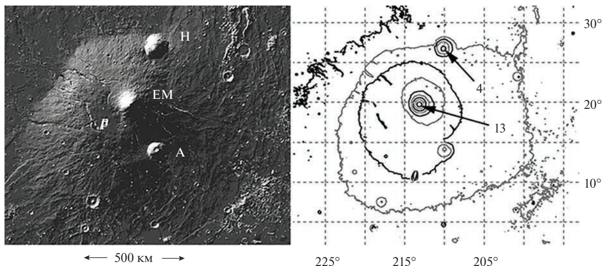
Рис. 5. Космические изображения и карта МГС гора Элизий. EM — конус в. Элизий, H и A — частично погребенные конусы куполов-вулканов Гекаты и Альбор. Ниже горизонтали 0 км — горизонтали с отметками –1 и –2 км. Диаметр кратера в. Элизий равен 14 км, глубина – 0.1 км, по [Plescia, 2004].
