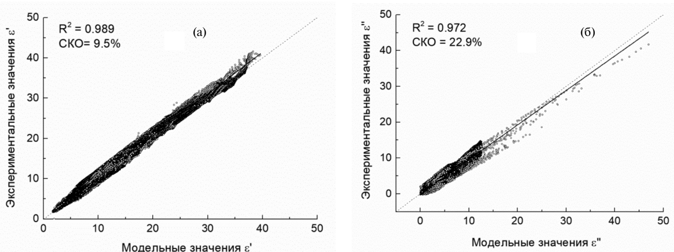
Рис. 7. Зависимость экспериментальных данных от полученных с помощью разработанной ОРДМВП для диэлектрической проницаемости (а), \varepsilon' , и коэффициента потерь (б), \varepsilon'' , для всех почв при всех влажностях образцов и температурах измерения. Символы – экспериментальные данные, сплошная линия – линейная аппроксимация, пунктирная линия – биссектриса.
