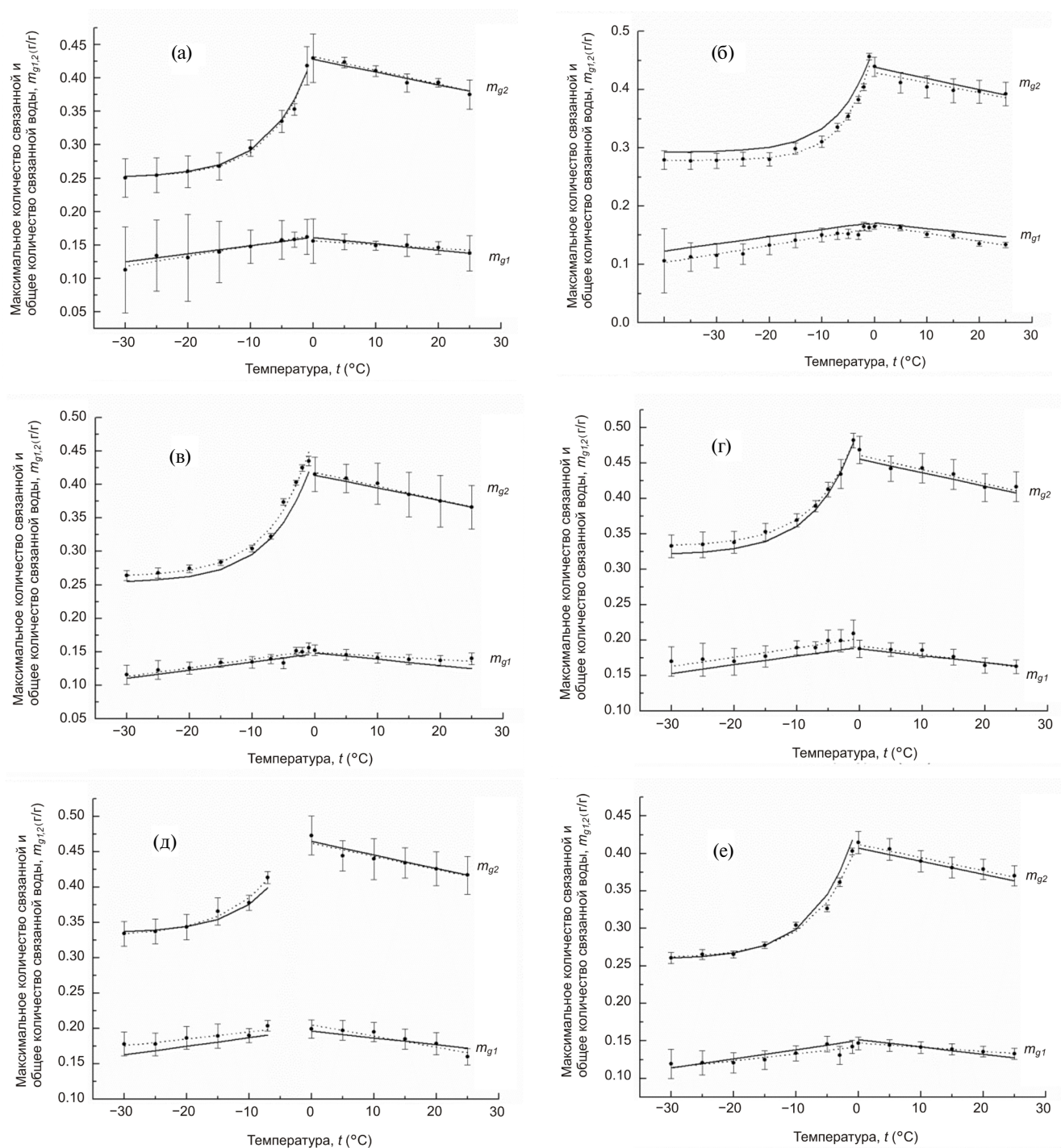
Рис. 1. Температурные зависимости предельных значений содержания прочносвязанной и рыхлосвязанной воды в почве (символы — экспериментальные данные; сплошная линия — расчет по модели; пунктирная линия — аппроксимация экспериментальных данных). Образец № 1 — (а), № 2 — (б), № 3 — (в), № 4 — (г), № 5 — (д), № 6 — (е).
