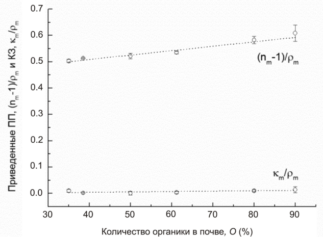
Рис. 2. Зависимость приведенного ПП, (n_m - 1)/\rho_m , и приведенного НКЗ, \kappa_m/\rho_m , от количества органического вещества в почве.
