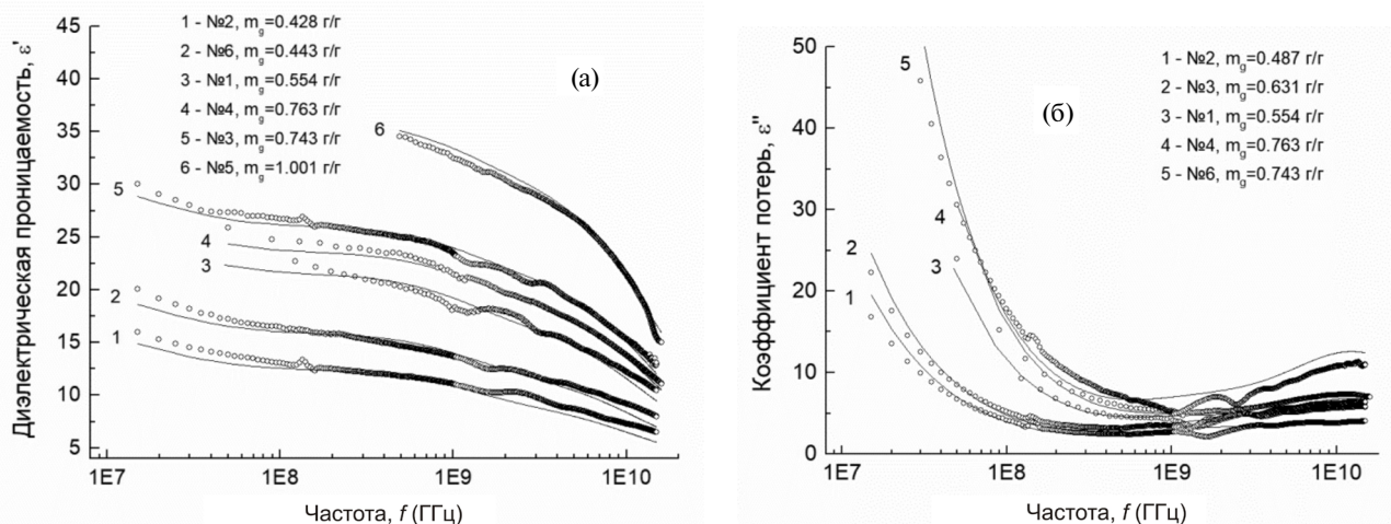
Рис. 3. Спектры диэлектрической проницаемости (а), \epsilon' и коэффициента потерь (б), \epsilon'' для различных почв и влажностей при температуре t = 20^\circ\text{C} . Экспериментальные данные – символы, результат аппроксимации – линии.
