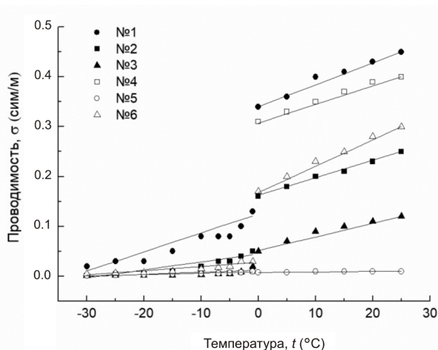
Рис. 6. Проводимость как функция температуры. Символы — данные полученные из измерений, линии — соответствующие им аппроксимации для свободной воды ( t > 0 ), \sigma_w , и влажного льда ( t < 0 ), \sigma_i , для всех исследуемых почв.
