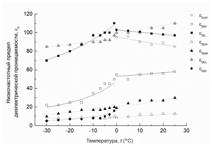
Рис. 4. Низкочастотный предел ДП как функция температуры. Символы — данные полученные из измерений, линии — соответствующие им аппроксимации, для связанной воды, \epsilon_{0bQ} , переходной связанной воды, \epsilon_{0iQ} , несвязанной воды, \epsilon_{0uQ} и влажного льда, \epsilon_{0iQ} , для высоко- ( Q = H ), средне- ( Q = M ), и низкочастотной ( Q = L ) релаксации.
