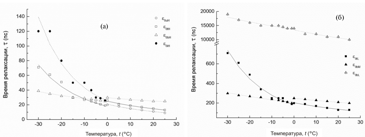
Рис. 5. Время релаксации как функция температуры. Символы — данные полученные из измерений, линии — соответствующие им аппроксимации, для связанной воды, \tau_{0bQ} , переходной связанной воды, \tau_{0iQ} , несвязанной воды, \epsilon_{0uQ} и влажного льда, \epsilon_{0iQ} , для высоко- ( Q = H ), средне- ( Q = M ), и низкочастотной ( Q = L ) релаксации.
