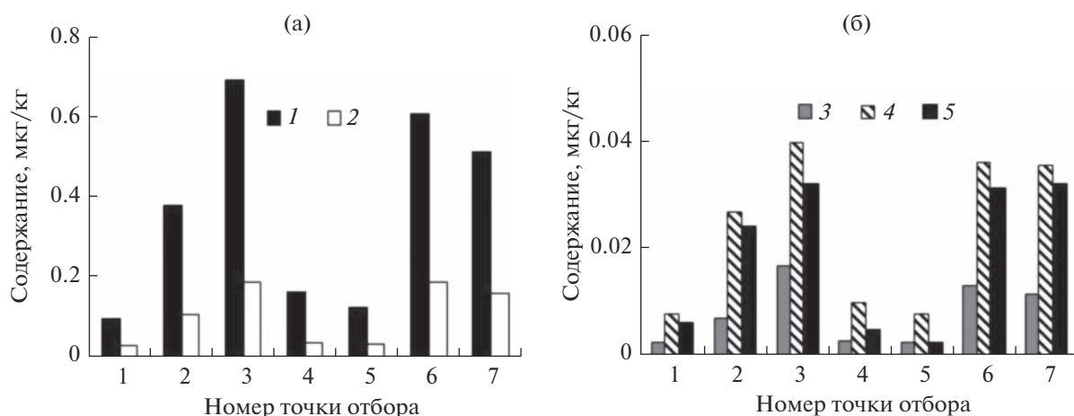
Рис. 8. Содержание пентаароматических УВ в ДО: 1 – трифенилен, 2 – метилбензантрацен, 3 – бензфлуорант렌, 4 – метилхризен, 5 – диметилбензантрацен.
