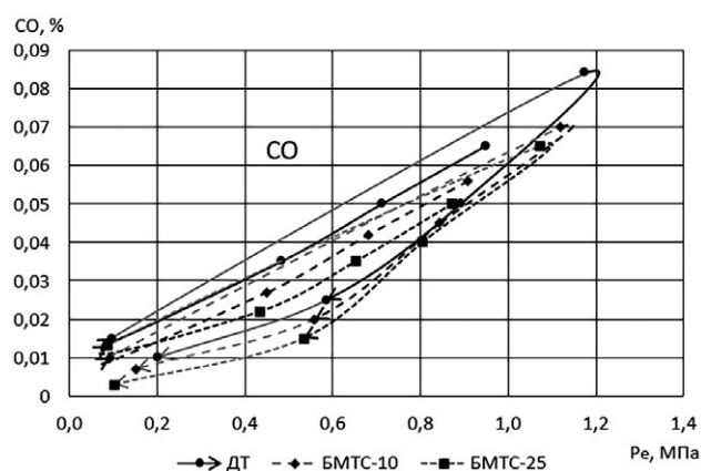
Рис. 3. Нагрузочные характеристики испытательного цикла согласно Правилам ООН №96 (02) (концентрация монооксида углерода CO).
