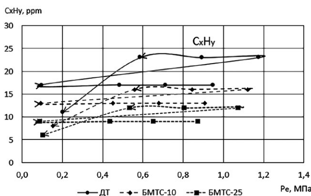
Рис. 5. Нагрузочные характеристики испытательного цикла согласно Правилам ООН №96 (02) (концентрация углеводородов C_xH_y ).
