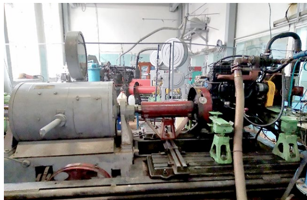
Рис. 1. Электротормозной стенд RAPIDO SAK N670 с балансирующей маятниковой машиной.
