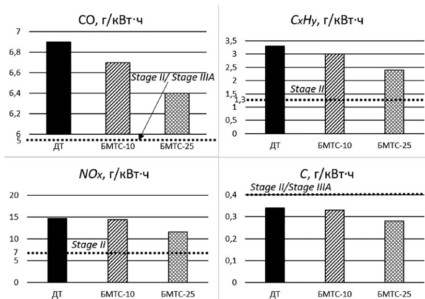
Рис. 7. Суммарные значения удельного выброса токсичных веществ за весь испытательный цикл. Fig. 7. Total values of specific emission of toxic substances for the entire test cycle.
