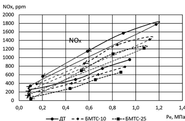
Рис. 6. Нагрузочные характеристики испытательного цикла согласно Правилам ООН №96 (2) (концентрация оксидов азота NO_x ).
