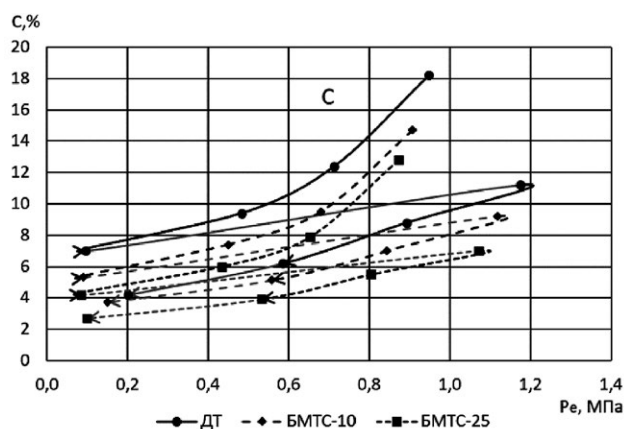
Рис. 4. Нагрузочные характеристики испытательного цикла согласно Правилам ООН №96 (02) (концентрация углерода С).
