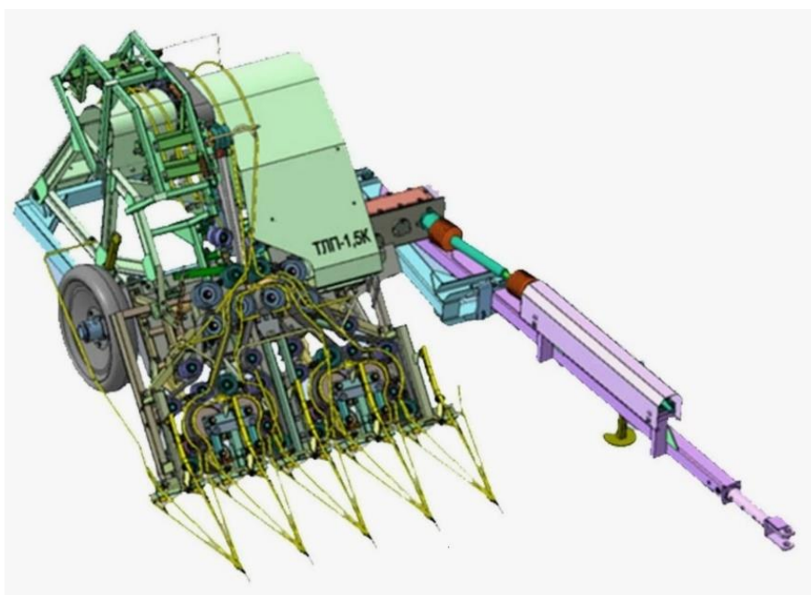
Рис. 4. Прицепная теребилка льна ТЛП-1,5К.
