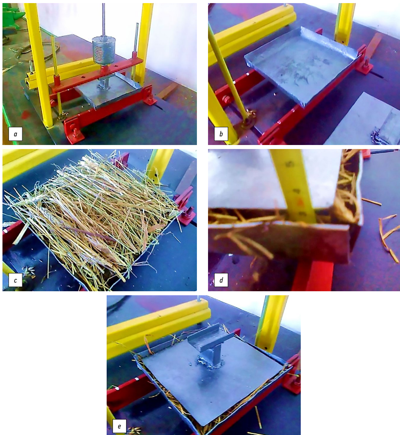
Рис. 2. Исследование плющения соломы: a — лабораторная установка; b — ёмкость для закладки соломы; c — закладка стеблей; d — воздействие начальной силы; e — измерение уплотнения.
