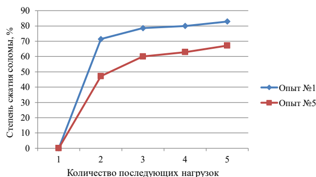
Рис. 4. Степень сжатия соломы.
