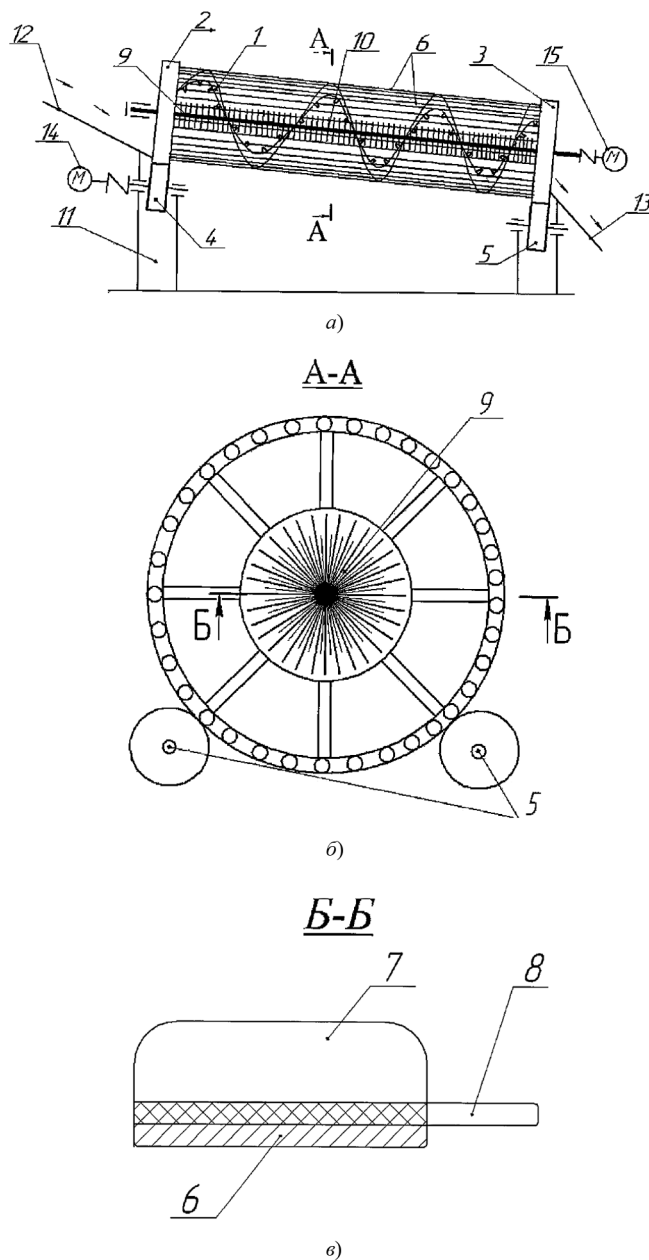
Рис. 2. Устройство для очистки корнеклубнеплодов от примесей [8]:
