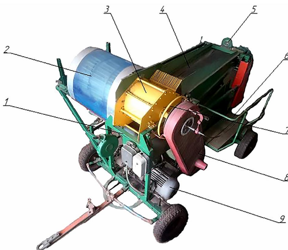
Рис. 2. Молотилка АРПМСУ: 1 — основание; 2 — молотильно-сепарирующее устройство; 3 — шнек-питатель; 4 — подающий транспортер; 5 — тахометр контроля оборотов ротора; 6 — площадка оператора; 7 — штурвал регулирования оборотов ротора; 8 — защитный кожух клиноременного вариатора; 9 — электродвигатель.
