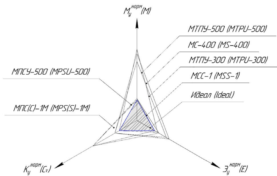
Рис. 1. Многокритериальная оценочная модель исследуемых молотилок серийного производства. Fig. 1. Multi-criteria evaluation model of the studied in-series threshers (according to specific criteria of energy intensity: E , material intensity: M , and versatility coefficient: C_v ).
