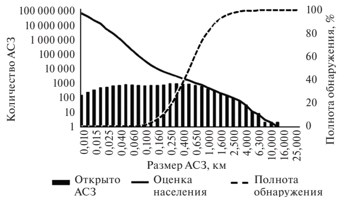
Рис. 3. Полнота обнаружения АСЗ (штриховая линия) и прогнозируемое распределение популяции АСЗ по размерам (сплошная линия); количество известных АСЗ (тёмные столбцы) в интервале размеров (данные NASA)
