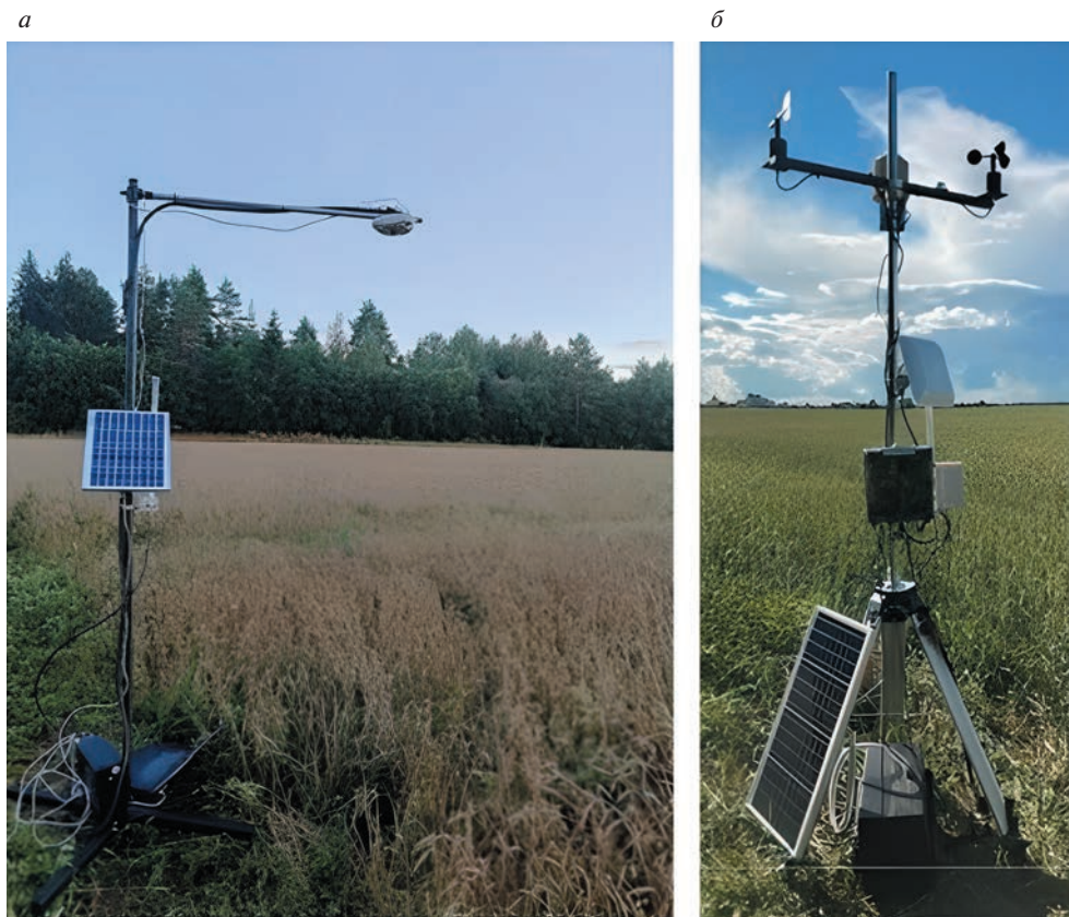
Рис. 1. Сенсорный узел (а), оснащённый оптическим датчиком для мониторинга состояния растительности, и базовая станция с интернет-каналом передачи данных для мониторинга метеорологических параметров (б)
