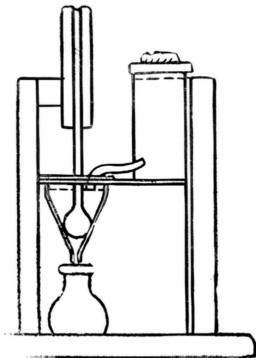
Рис. 4. Прибор Ломоносова для определения вязкости жидкостей [12, с. 75]
