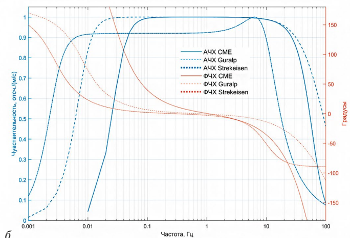
Рис. 2. Макет вмораживаемого геогидроакустического информационно-измерительного буя (а) и амплитудно-частотные и фазочастотные характеристики молекулярно-электронных сейсмоприёмников (СМЕ-4211V) и эталонных маятниковых сейсмоприёмников Guralp (CMG-3ESP) и Streckeisen (STS-1V/VBB) (б)
