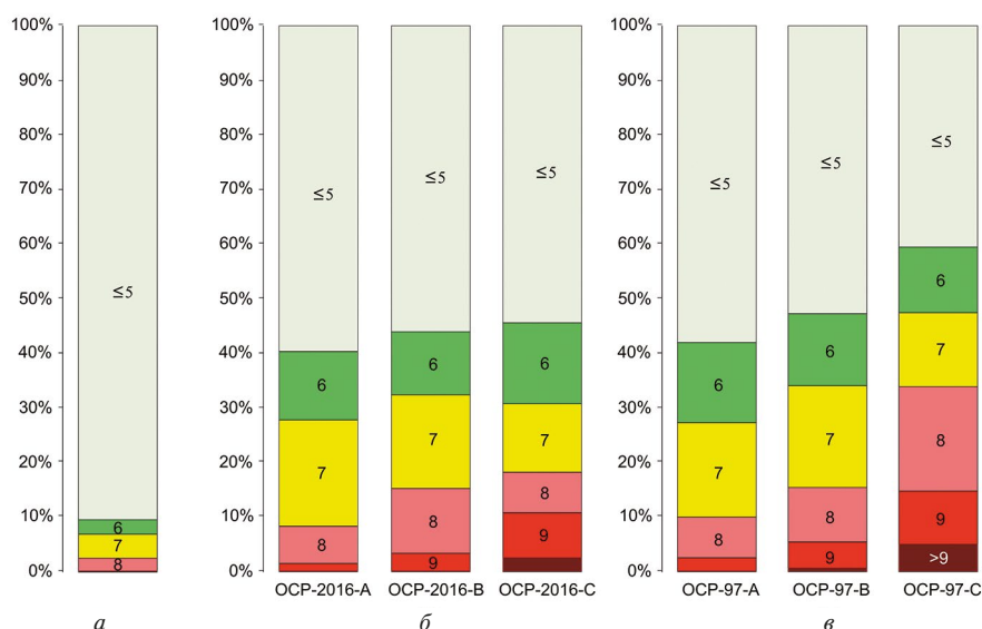
Рис. 1. Сопоставление площадей разной балльности на картах ОСП-97 и ОСП-2016 и реальных землетрясений a – доли суммарной площади теоретических изосейст 6, 7, 8 и 9 баллов от землетрясений в 1997–2022 гг., умноженные на 20; б – доли площадей зон разной балльности (6 и более) на картах ОСП-2016; в – на картах ОСП-97; площадь территории России принята за 100%; карты с пометкой “А” отвечает вероятности 0.1 превышения соответствующей интенсивности за 50 лет, карты “В” – 0.05, карты “С” – 0.01
