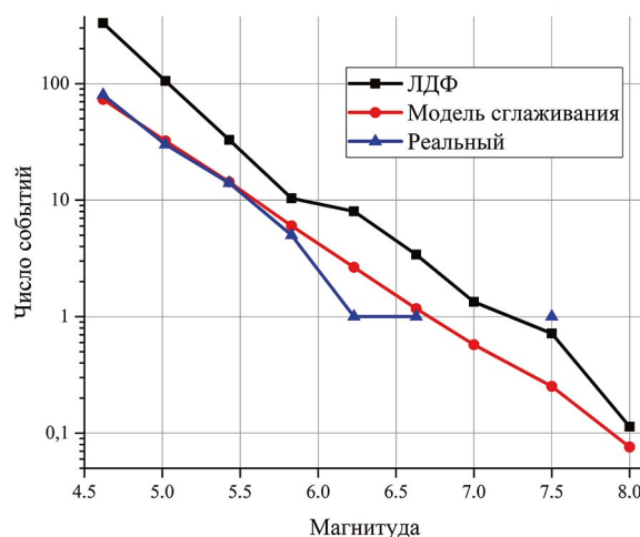
Рис. 3. Магнитудно-частотное распределение для реального каталога землетрясений восточного сектора российской Арктики за 1982–2020 гг. (треугольники) и ЛДФ-модели, приведённой к эквивалентному периоду 39 лет (квадраты)
