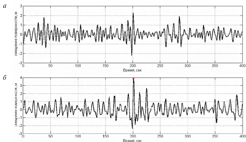
Рис. 9. Примеры аномально больших волн (волн-убийц), зарегистрированных у мыса Свободный:
