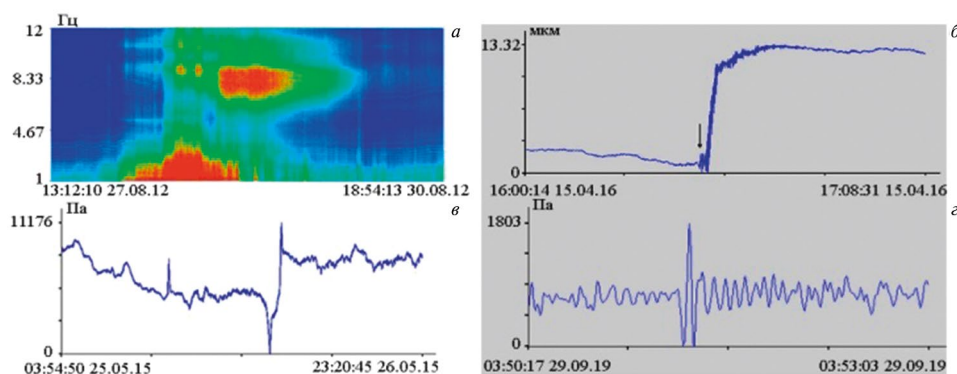
Рис. 2. Фрагменты записей и динамическая спектрограмма лазерно-интерференционных приборов:
