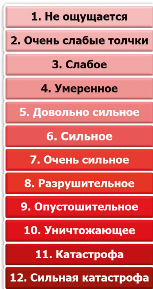
Рис. 3. 12-балльная шкала Медведева—Шпонхойера—Карника (MSK-64). Общая характеристика зон балльности
