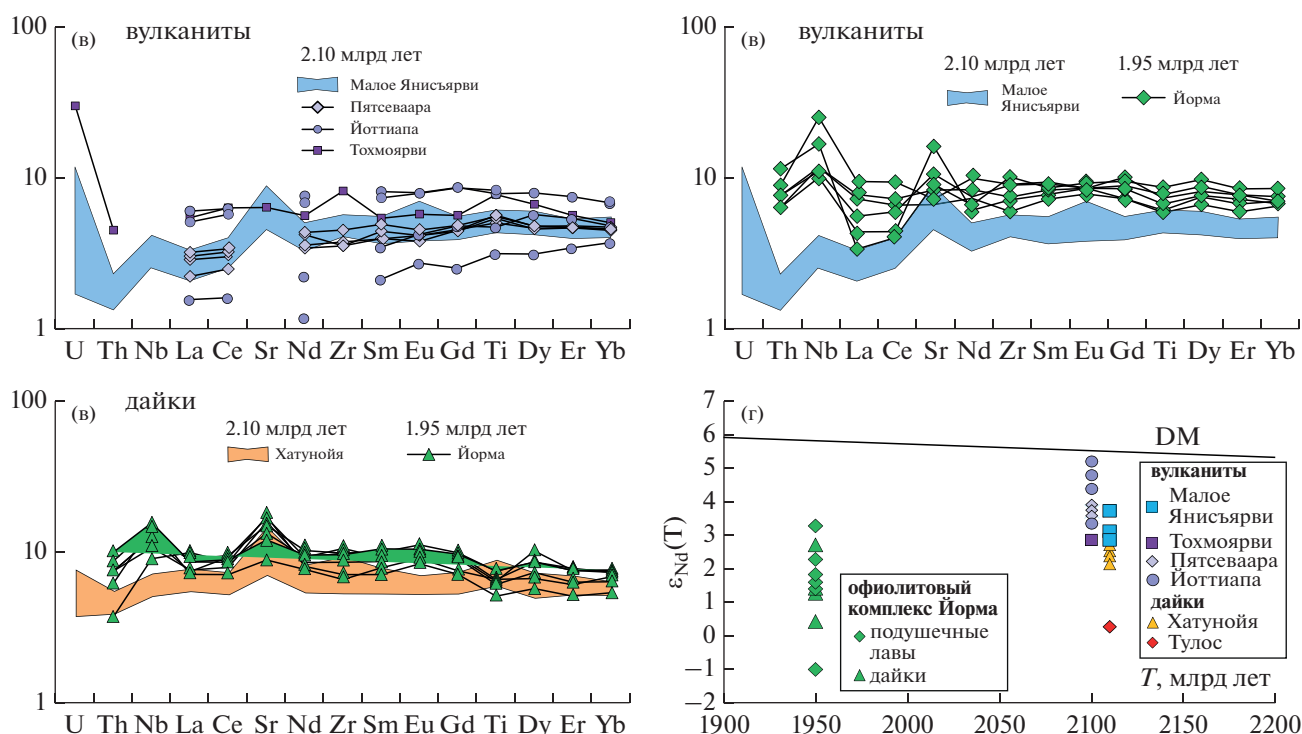
Рис. 9. Сравнение геохимических и изотопных характеристик вулканитов и даек деплетированных толеитов с возрастaми 2.10 и 1.95 млрд лет из западной части Карельского кратона (Раахе-Ладожская зона). (а–в) – мультиэлементные диаграммы (нормировано к примитивной мантии: Wenderpohl, Hartmann, 1994): (а) – вулканиты с возрастaми 2.10 млрд лет из участков Малое Янисъярви (это исследование), Пятсеваара (Матреничев, Матреничев, 2010), Йоттиапа (Nuhma et al., 1990) и Тохмоярви (Nykänen et al., 1994); (б) – вулканиты с возрастaми 2.10 млрд лет участка Малое Янисъярви и вулканиты с возрастaми 1.95 млрд лет из комплекса Йорма (Peltonen et al., 1996); (в) – дайки с возрастaми 2.10 млрд лет участка Хатунойя и дайки с возрастaми 1.95 млрд лет из комплекса Йорма (Peltonen et al., 1996); (г) – диаграмма \epsilon_{Nd}(T) –возраст для вулканитов и даек с возрастaми 2.10 и 1.95 млрд лет из Раахе-Ладожской зоны по нашим данным и из работ (Nuhma, 1986; Nuhma et al., 1990; Nykänen et al., 1994; Peltonen et al., 1996; Матреничев, Матреничев, 2010).
