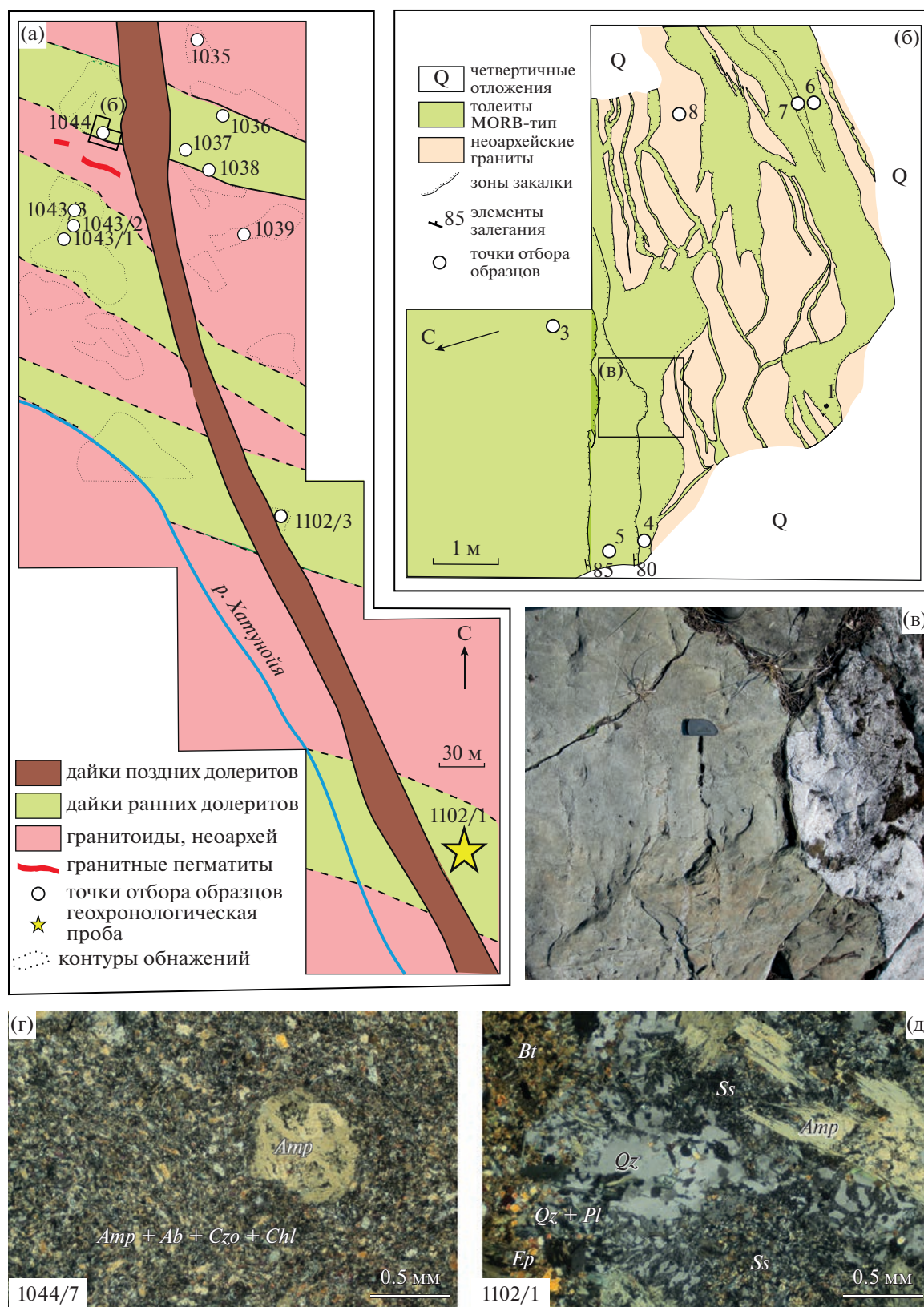
Рис. 3. Геологическое строение и петрографические характеристики пород на участке Хатунойя: геологическая схема соотношения ранних и поздних даек на участке Хатунойя (а) и схема внутреннего строения ранних даек (б); макро-скопические (в) и микроскопические (г) фотографии (XPL), иллюстрирующие зоны закалок внутри тел ранних даек на участке Хатунойя; (д) микрофото (XPL) образца датированного габбро-пегматита. Ss – агрегат сосюрита.
