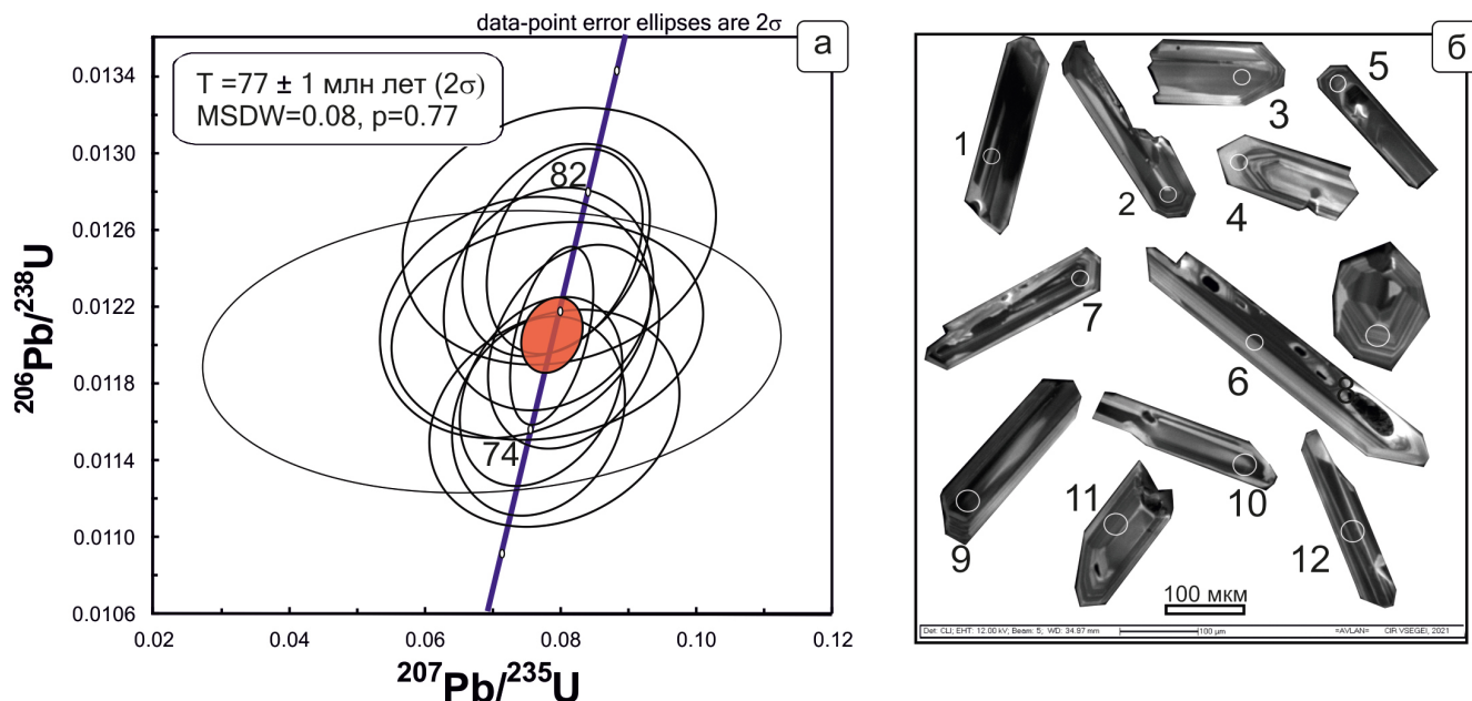
Рис. 16. Диаграмма с конкордией результатов U–Pb датирования циркона из киловых пеплов Крыма (а) и изображение кристаллов датированных цирконов в катодолуминисцентном излучении (б). Номера соответствуют точкам в табл. 1.
