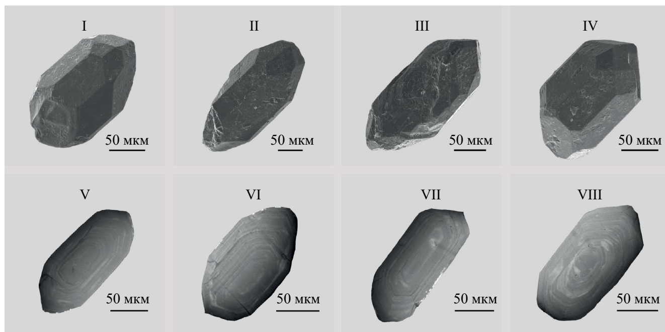
Рис. 6. Микрофотографии кристаллов циркона из метадациита (пр. 13/14) Мегриарвинской структуры, выполненные на СЭМ TESCAN VEGA 3 в режимах вторичных электронов (I–IV) и катодолуминесценции (V–VIII).
