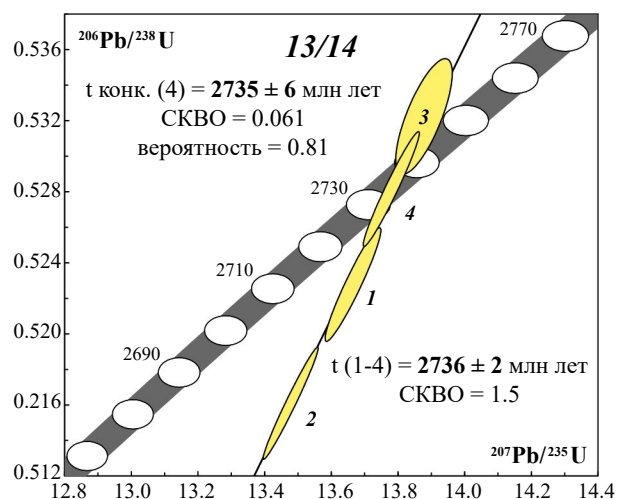
Рис. 7. Диаграмма с конкордией для циркона из метадациита (проба 13/14) Мегриарвинской структуры. Номера точек соответствуют номерам в табл. 2.
