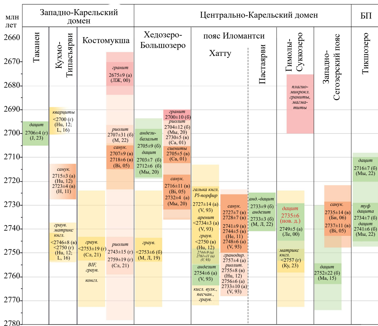
Рис. 3. Схема корреляции U–Pb (по циркону) геохронологических данных для неогархейских вулканических и осадочных пород гимольского надгоризонта (левый столбец); для субвулканических и интрузивных пород (правый столбец), полученных: (а) классическим методом (TIMS), (б) SIMS, SHRIMP II, (в) SIMS, Nordsim, (г) LA-ICP-MS.
