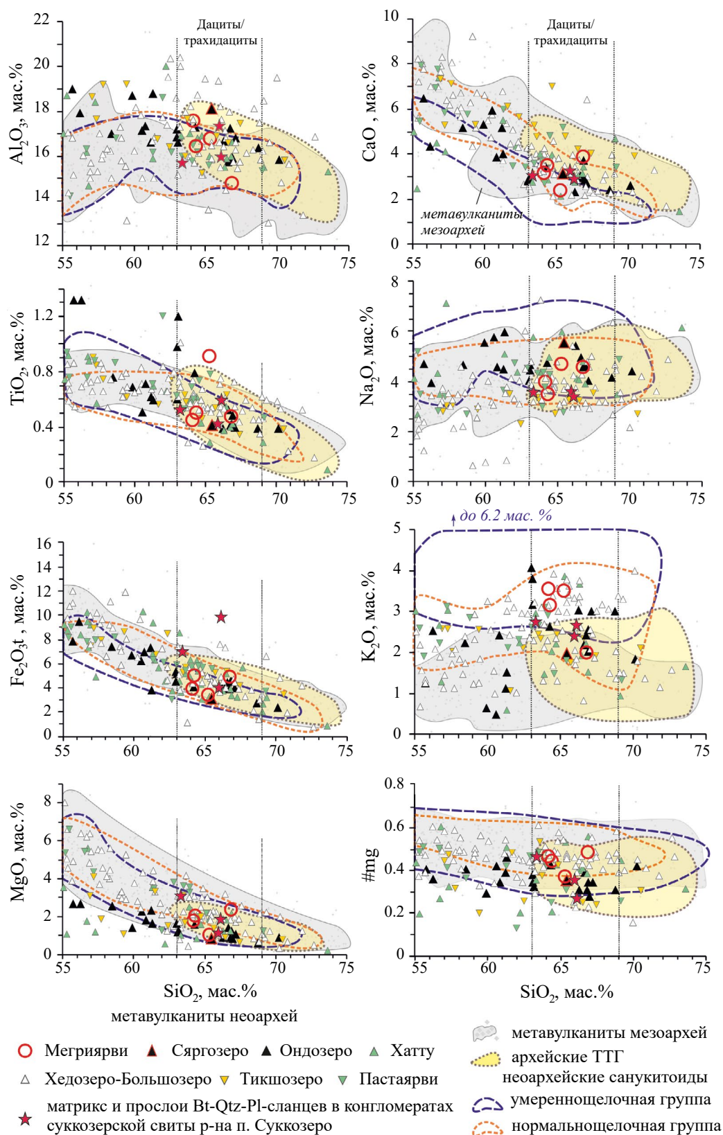
Рис. 8. Соотношение содержаний главных элементов и магнезиальности относительно \text{SiO}_2 для неоархейских метавулканитов среднекислого состава Центрально-Карельского домена и Тикшозерского пояса. Для сравнения показаны поля составов архейских пород Карельской провинции: мезоархейских вулканитов среднекислого состава, архейских ТТГ и санукитоидов Карельской провинции. Источники данных те же, что и на рис. 5.
