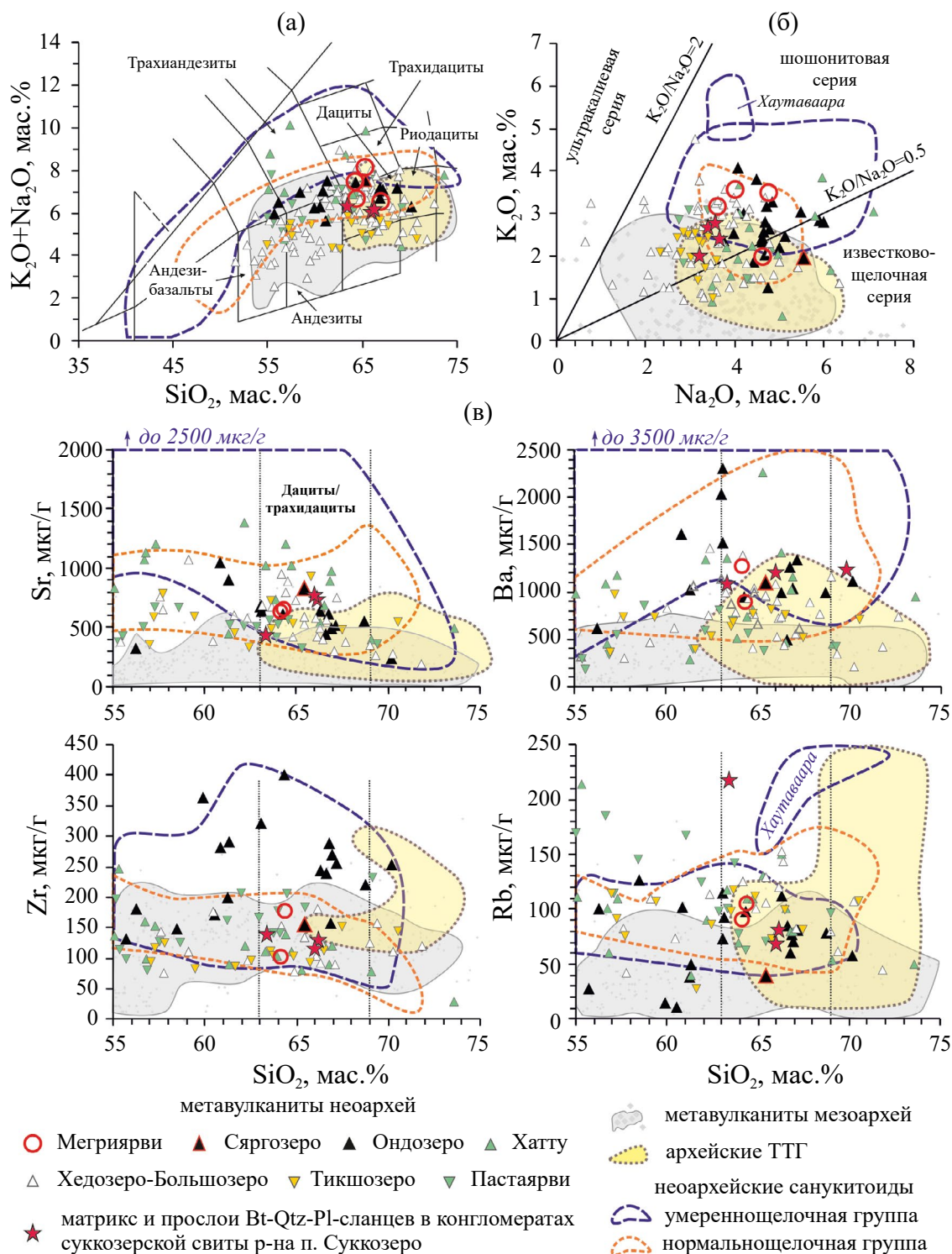
Рис. 5. Парные диаграммы, показывающие геохимические особенности метадациитов Мегриярви в сравнении с неогархейскими метавулканиитами других зеленокаменных структур Центрально-Карельского домена и Тикшозерского пояса, а также с полями составов архейских пород Карельской провинции: мезогархейских вулканиитов среднекислого состава, архейских ТТГ и санукитоидов.
