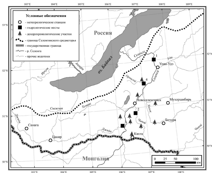
Рис. 1. Территория исследования и расположение на ней метеорологических станций, гидрологических постов (1 — р. Селенга—рзд. Мостовой; 2 — р.Чикой—с. Поворот; 3 — р. Джиды—с. Джиды; 4 — р. Оронгой—Оронгойский мост) и дендрохронологических участков.
