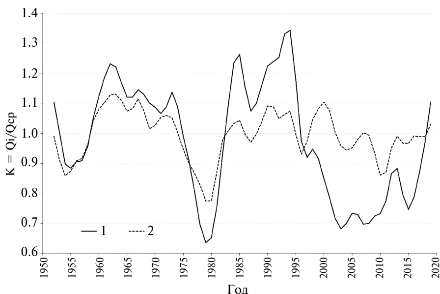
Рис. 5. Многолетние изменения годового стока р. Селенги у рзд. Мостового (1) и годовых сумм атмосферных осадков, осредненных по территории Селенгинского среднегорья (2), сглаженных с помощью пятилетнего скользящего осреднения.
