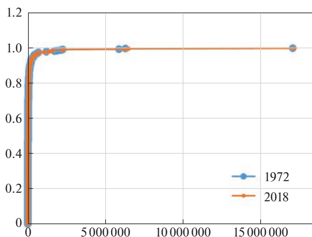
Рис. 6. Пример сопоставления распределений площадей озер за разные сроки в пределах озерно-термокарстовых равнин (участок 20).
