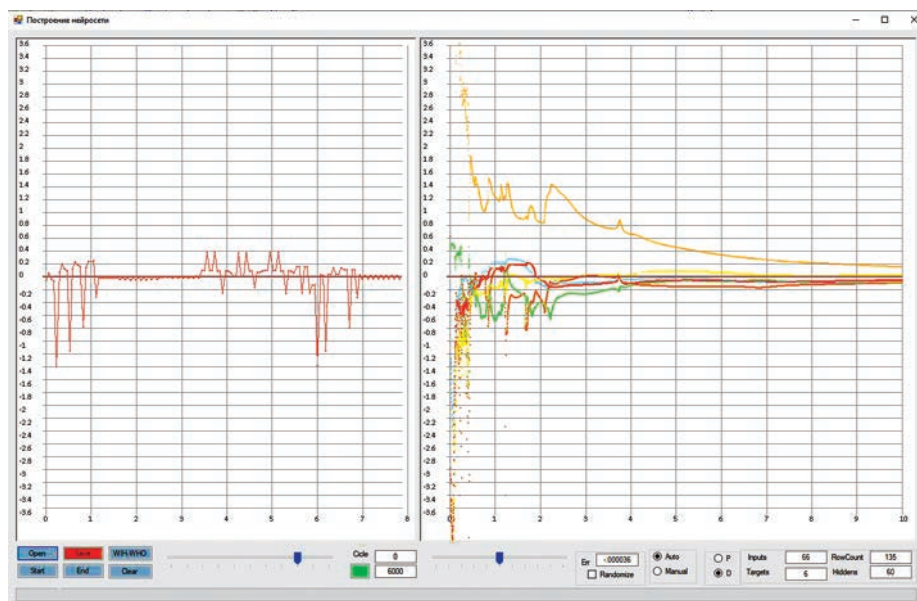
Рис. 6. Построение нейросети.
