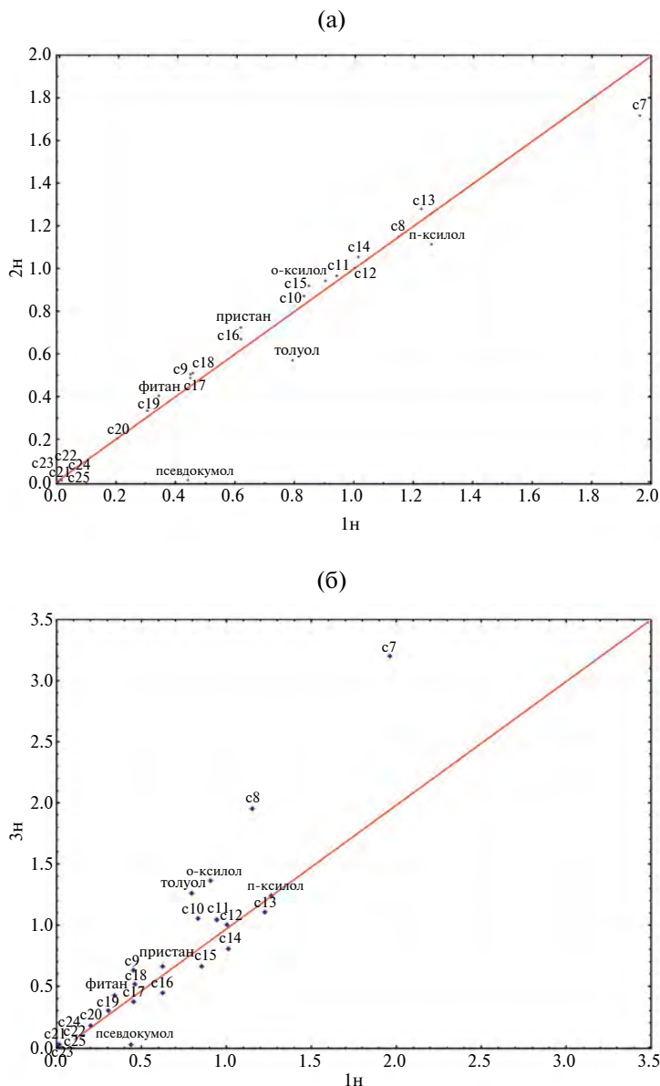
Рис. 5. Сопоставление нормированных концентраций углеводородов в пробах: а — 1n и 2n , б — 1n и 3n .
