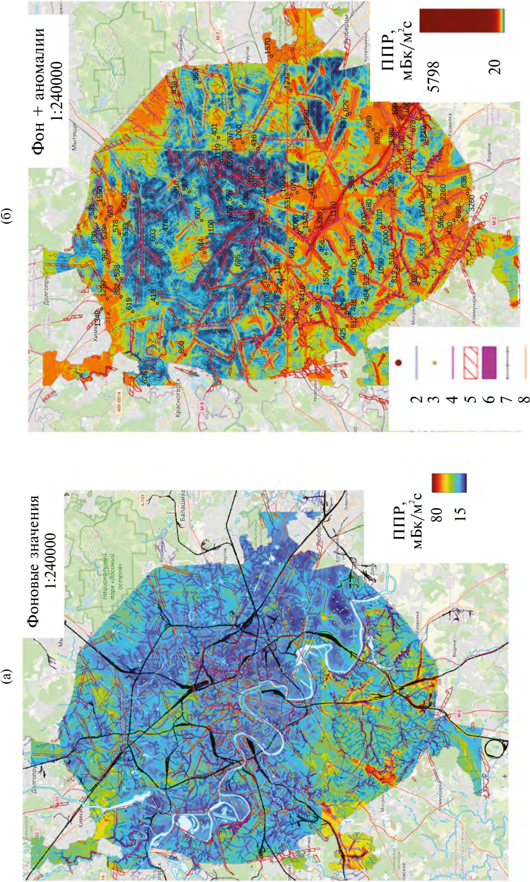
Рис. 3. Карта прогноза ППР, составленная с использованием: а – фоновых значений и алгоритма Random Forest; б – полного набора данных (аномальные и фоновые участки). Алгоритм Random Forest с квантильным цветовым масштабированием. Условные обозначения: 1 — участки с аномалиями ППР, 2 — тальвеги, 3 — участки с фоновыми значениями ППР, 4 — линейные зоны, 5 — геодинамически активные зоны, 6 — уклоны более 8°, 7 — железные дороги, 8 — линии метро.
