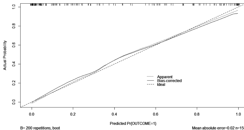
Рис. 5. Калибровочная кривая (КК) для модели исхода (Apparent – КК по оригинальному набору данных, Bias-corrected – КК, скорректированная на оптимизм, Ideal – идеальная КК)
