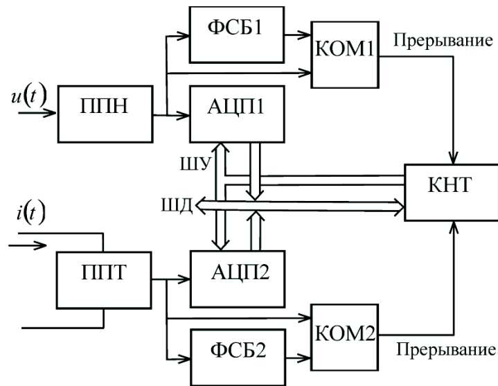
Рис. 2. Схема ИИС, реализующей метод
