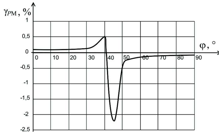
Рис. 3. График зависимости погрешности измерения АМ (РМ) от \varphi
