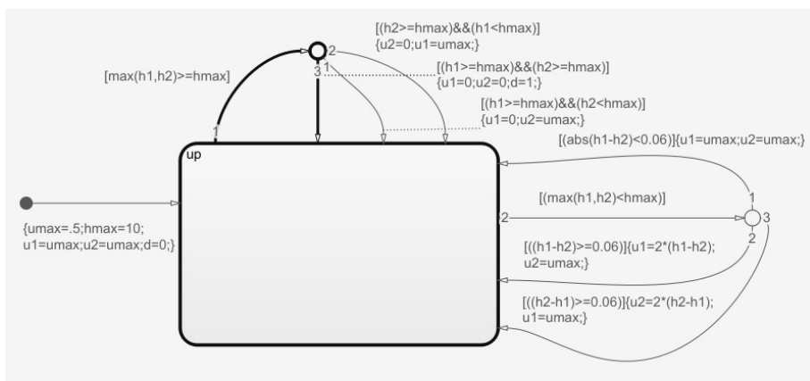
Рис. 7. Stateflow-диаграмма регулятора
