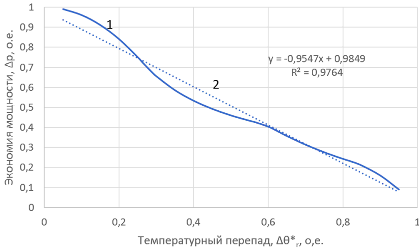
Рис. 4. Графики зависимости экономии мощности от требуемого температурного перепада: 1 – оптимальное комбинированное управление \Delta p_2(\Delta \theta_r^*) ; 2 – линейная аппроксимация \Delta p_2(\Delta \theta_r^*)
