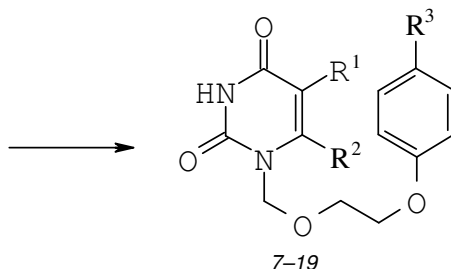
Схема. Синтез 1-[[2-(фенокси)этокси]метил]урацилов (7–19): R^1 = H, Me, Et, Br; R^2 = H, Me; R^3 = Me, Cl.
