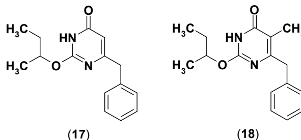
Рис. 9. 6-бензил-2-(1-метилпропокси)пиримидин-4(3Н)-он ( 17 ), 6-бензил-2-(1-метилпропокси)-5-метилпиримидин-4(3Н)-он ( 18 )
