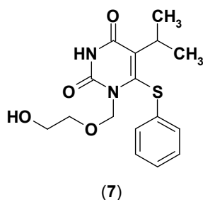
Рис. 3. 5-изопропил-1-[(2-гидроксиэтокси)метил]-6-(фенилтио)урацил
