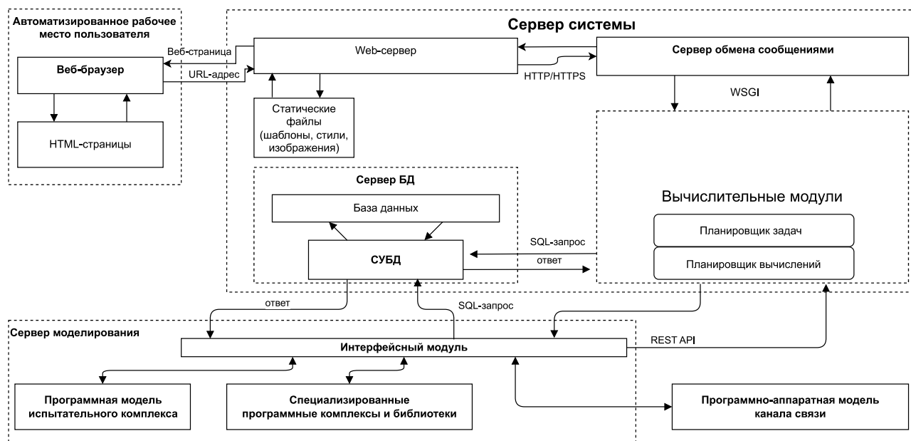
Рисунок 4. Архитектура PBC
