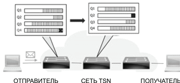
Рисунок 2. Распределенная схема динамического присвоения приоритетов на основе RL
