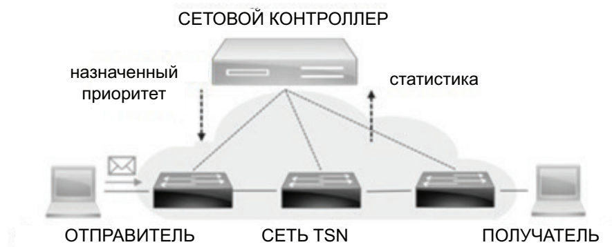
Рисунок 1. Централизованная схема динамического присвоения приоритетов
