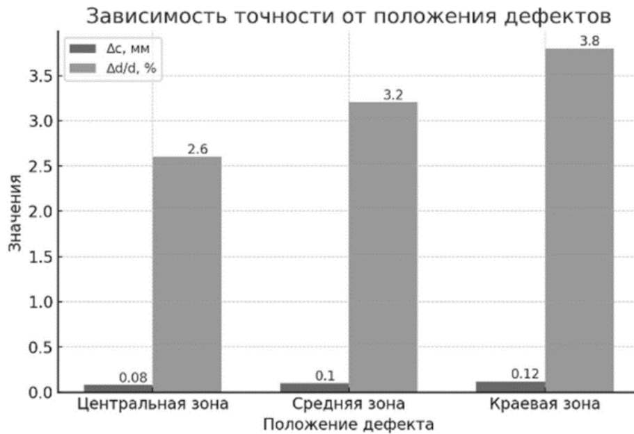
Рисунок 4. Зависимость точности от положения дефектов
