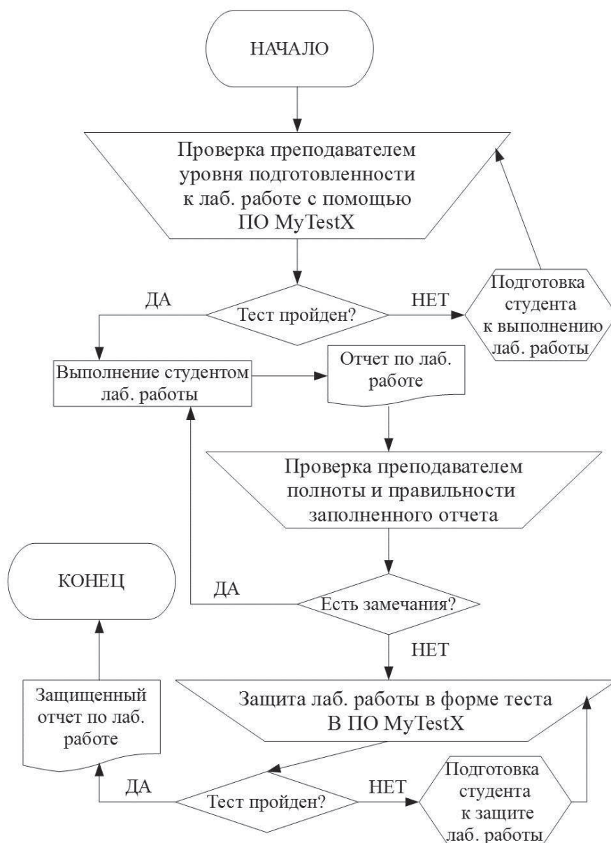
Рисунок 2. Схема выполнения лабораторной работы
