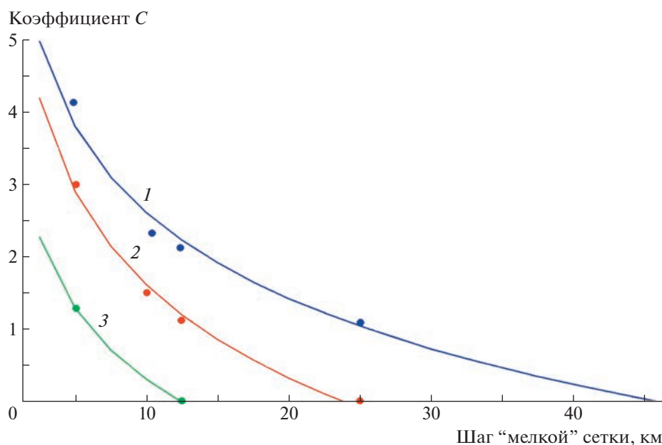
Рис. 4. Значения коэффициента C из табл. 2 (кружки) и соответствующие аппроксимации (кривые линии) при разных значениях размера "большой" ячейки. Коэффициент C связывает среднеквадратическое отклонение сжатия по группе "малых" ячеек и квадратный корень из среднего сжатия в "большой" ячейке: 1 – при шаге "грубой" сетки 50 км; 2 – при шаге "грубой" сетки 25 км; 3 – при шаге "грубой" сетки 12.5 км.
