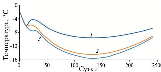
Рис. 4. Толщина снега (1), температура поверхности грунта (2) и воздуха (3) в районе метеостанции Баренцбург
