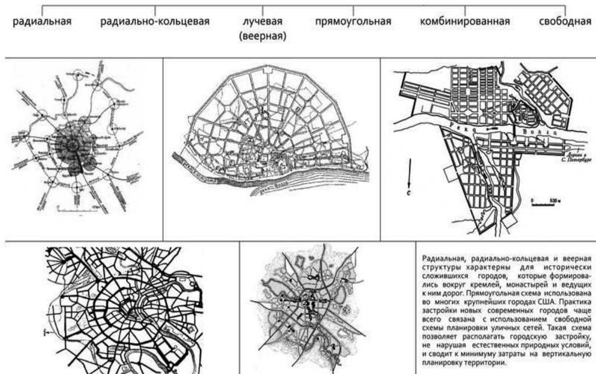
Рис. 3. Основные схемы построения уличных сетей городов мира
