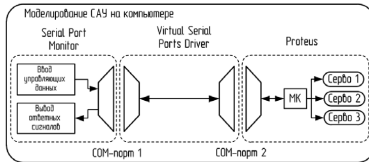
Рис. 3. Схема моделирования САУ на компьютере
